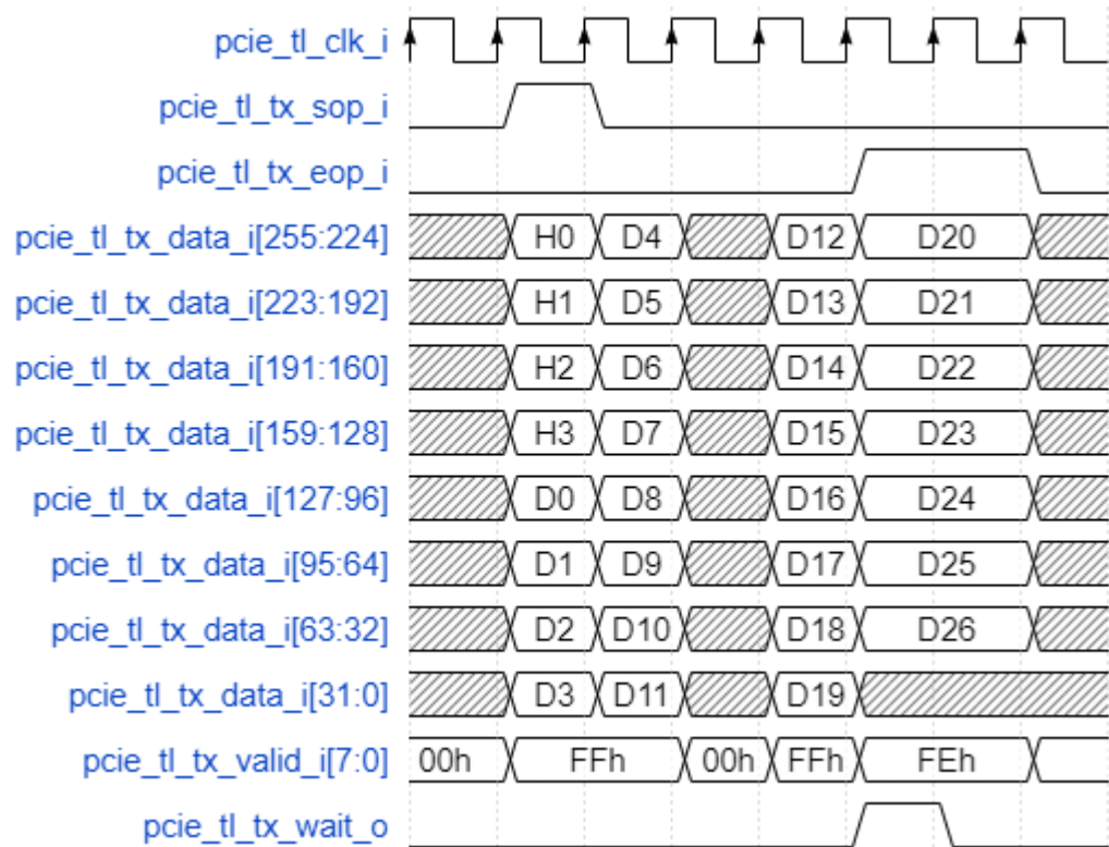
图 3-6 TLP 发送控制时序示例
