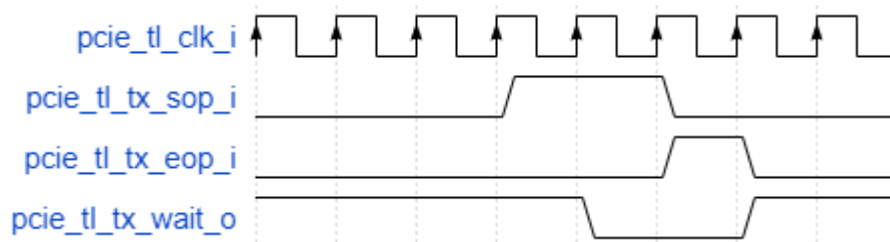
图 3-3 pcie_tl_tx_wait_i 与发送控制时序 1
