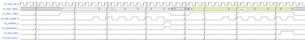
图 3-36 冲突时重发
