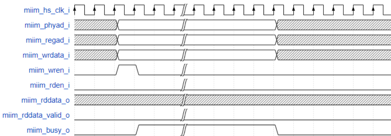
图 3-43 miim 写时序
