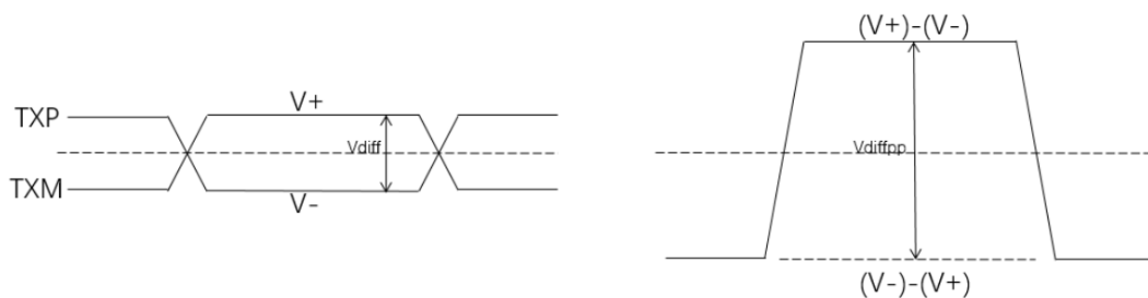
图 3-45 发送差分信号摆幅 V_{diffpp}
