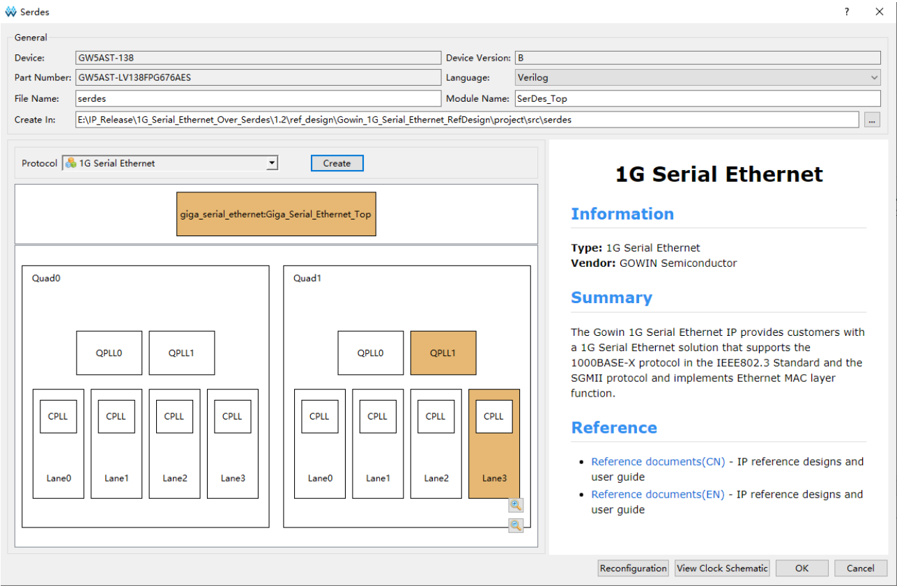
图 6-6 Serdes IP 配置界面显示 1G Serial Ethernet IP
