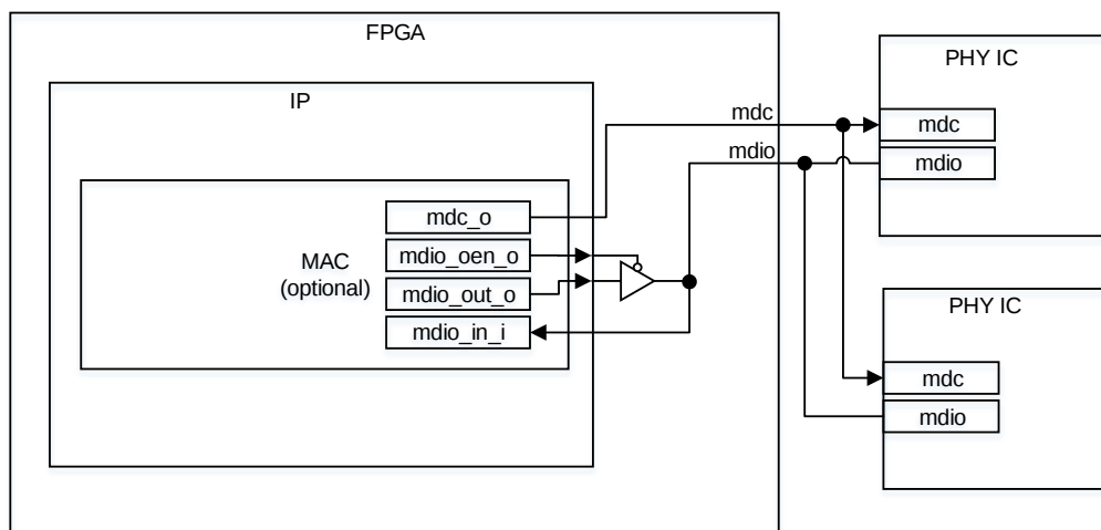
图 3-42 MDC、MDIO 连接示意图
