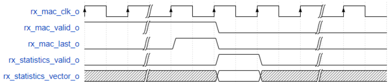
图 3-29 接收统计
