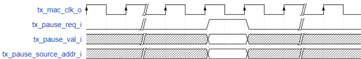
图 3-40 发送 Pause 帧
