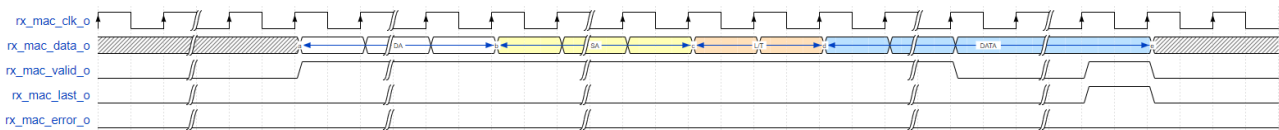
图 3-20 1000M 速率正常 MAC 帧接收
