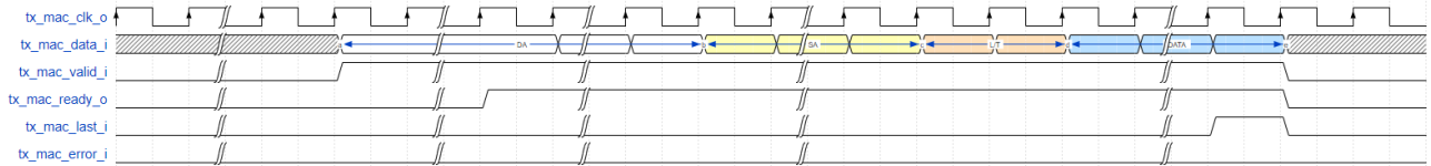
图 3-30 1000M 速率正常 MAC 帧发送
