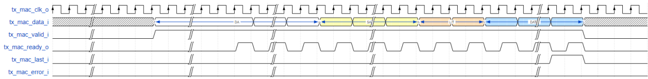
图 3-31 10M/100M 速率正常 MAC 帧发送
