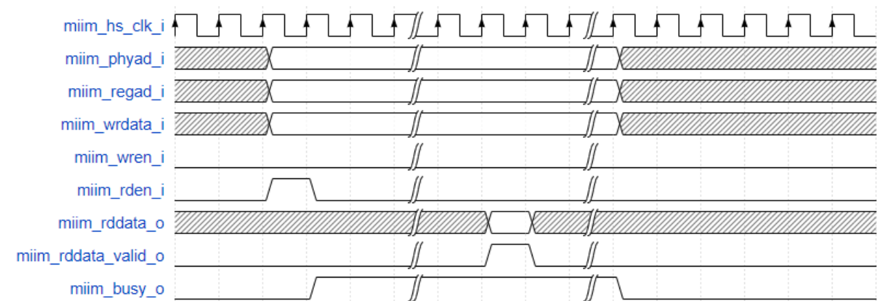
图 3-44 miim 读时序
