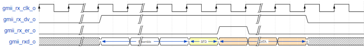
图 3-5 10M/100M 速率错误以太网帧接收
