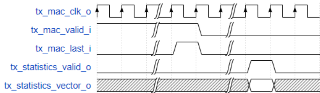
图 3-39 发送统计
