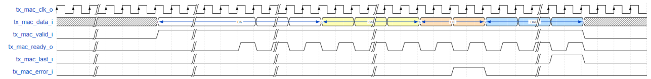
图 3-33 10M/100M 速率错误 MAC 帧发送
