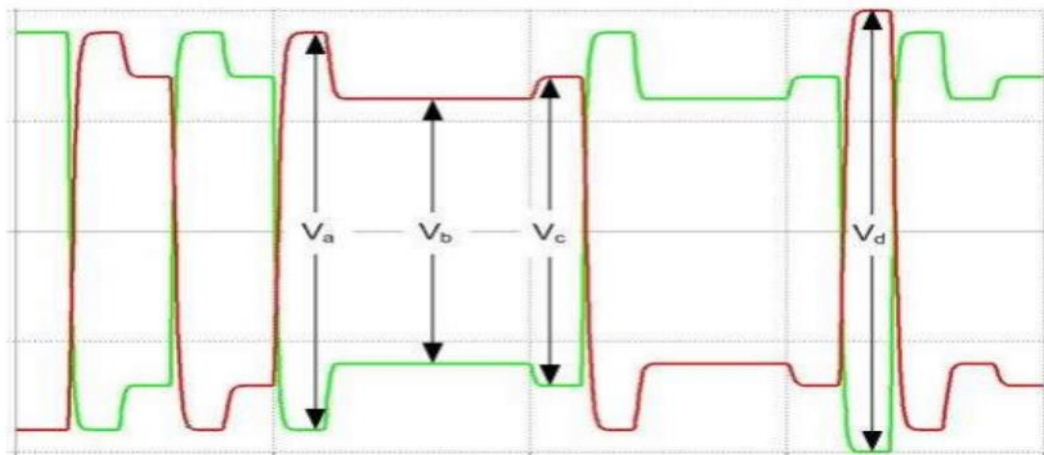
图 3-46 FFE TX 电压定义
