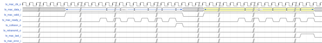
图 3-38 冲突时放弃重发（被动放弃）
