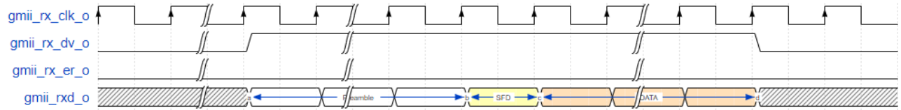
图 3-2 1000M 速率正常以太网接收
