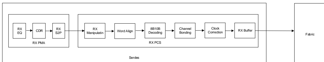
图 3-3 SerDes 接收部分
