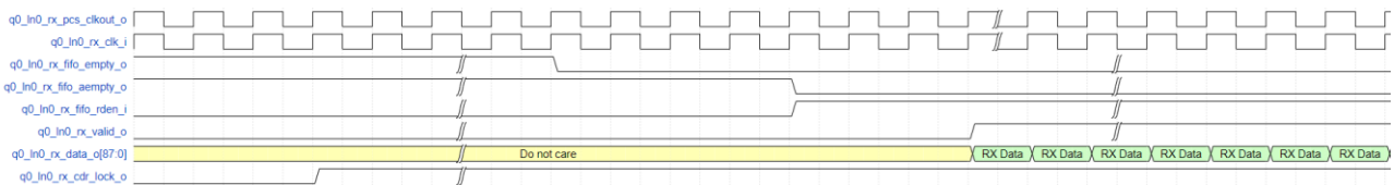
图 3-6 接收数据接口时序
