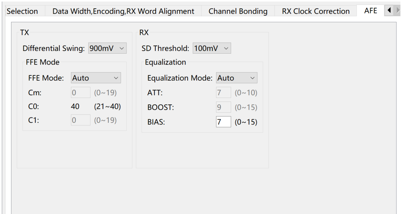
图 5-5 AFE 配置界面
