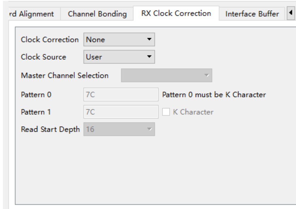
图 5-4 RX Clock Correction 配置界面
