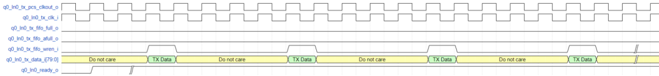
图 3-5 速率&lt;1Gbps 发送数据接口时序
