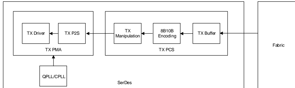
图 3-2 SerDes 发送部分
