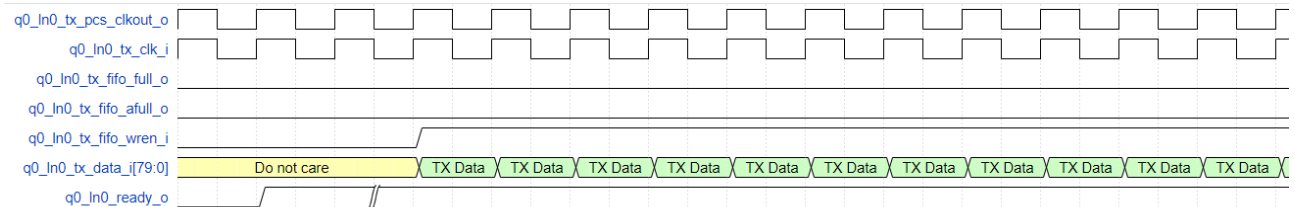
图 3-4 速率 \geq 1Gbps 发送数据接口时序
