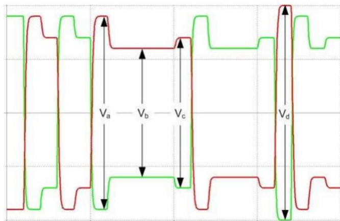
图 3-8 FFE TX 电压定义
