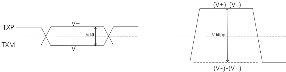
图 3-7 发送差分信号摆幅 V_{diffpp}
