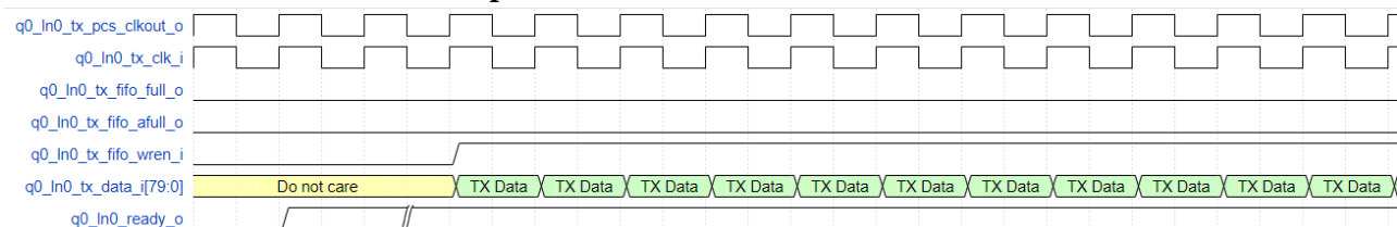
图 3-4 速率 \geq 1Gbps 发送数据接口时序
