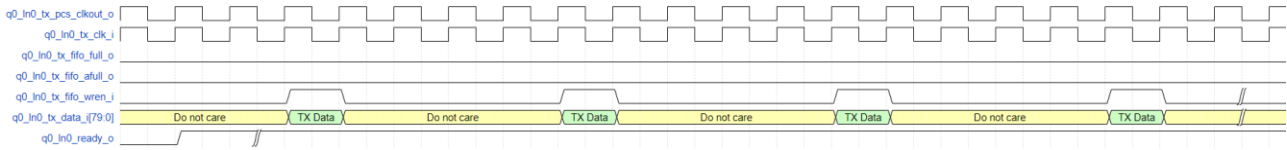
图 3-5 速率&lt;1Gbps 发送数据接口时序
