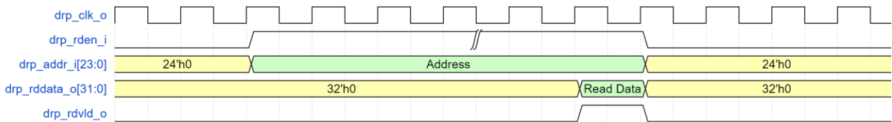
图 3-10 DRP 读操作时序图
