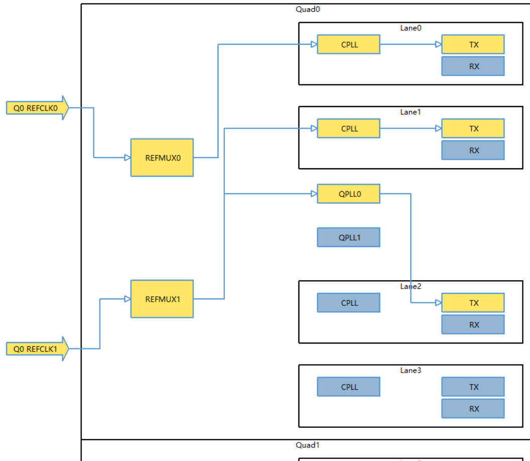
图 3-11 Clock Schematic
