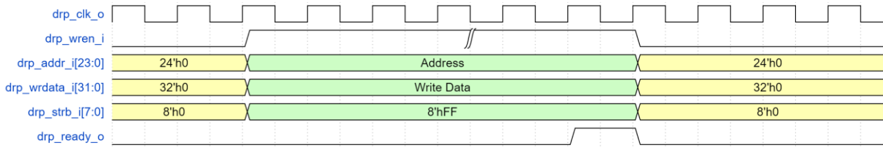
图 3-9 DRP 写操作时序图
