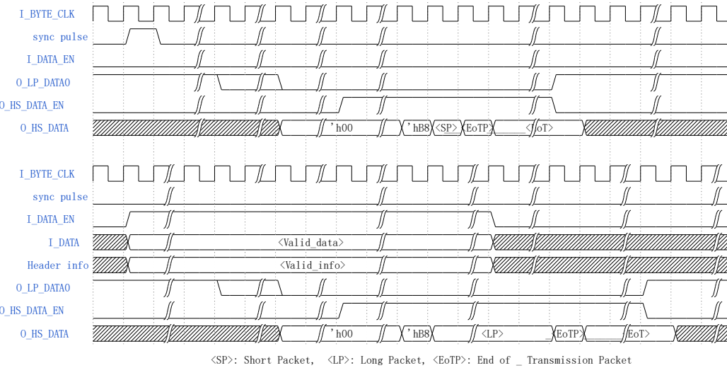
图 3-9 带 EoTP 的 DSI TX 时序示意图
