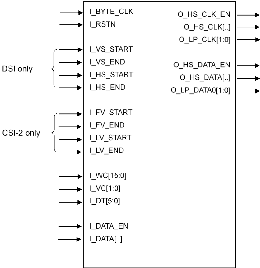
图 3-1 MIPI DSI/CSI-2 Transmitter IP 顶层框图
