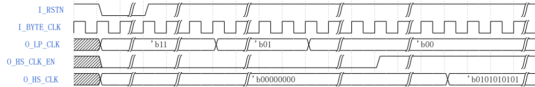
图 3-3 复位时序示意图
