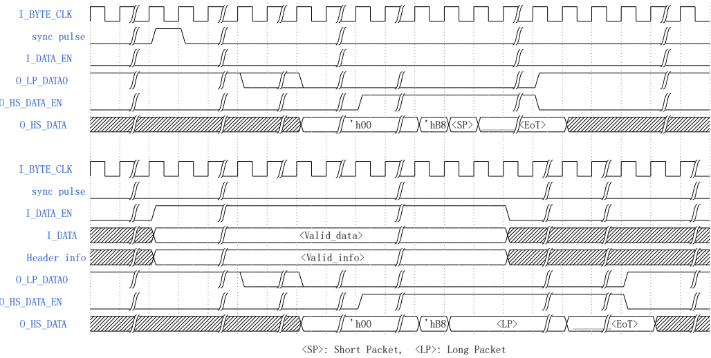
图 3-8 DSI/CSI-2 TX 时序示意图
