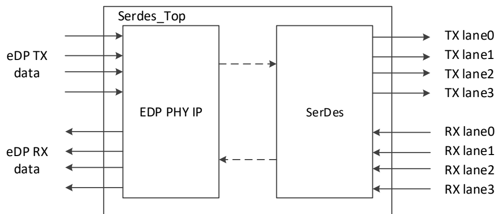
图 3-2 结构框图
