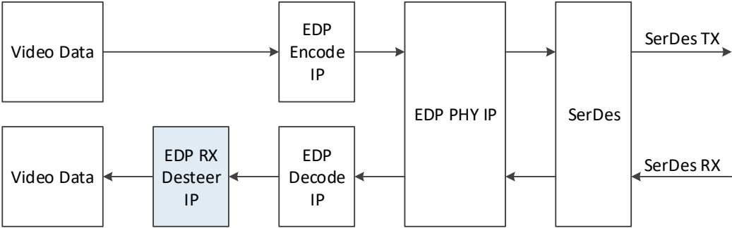
图 3-1 系统框图
