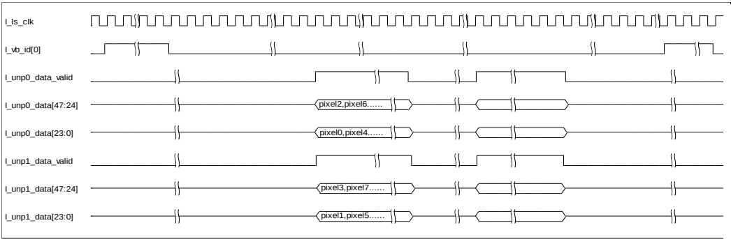
图 3-4 EDP RX Desteer 输入接口时序示意图(2 lanes)
