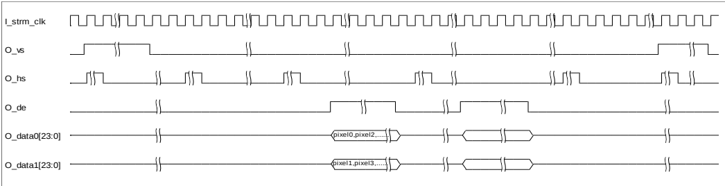
图 3-5 EDP RX Desteer 输出接口时序示意图(2lanes)
