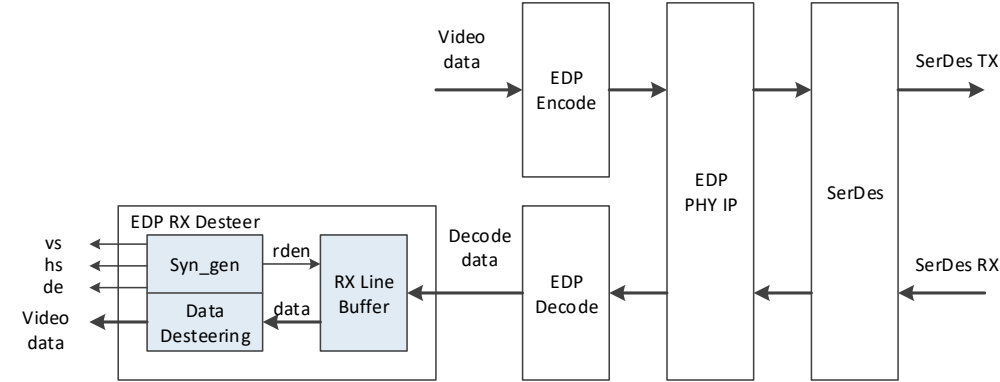
图 3-2 结构框图
