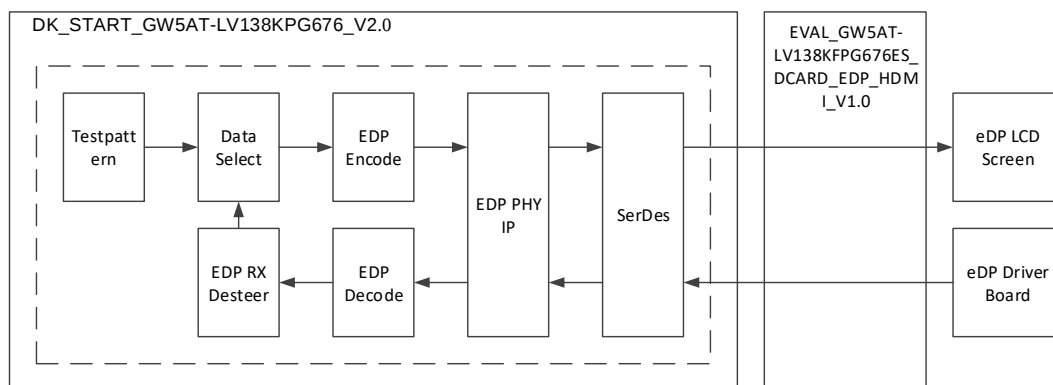
图 5-1 参考设计实例一基本结构框图
