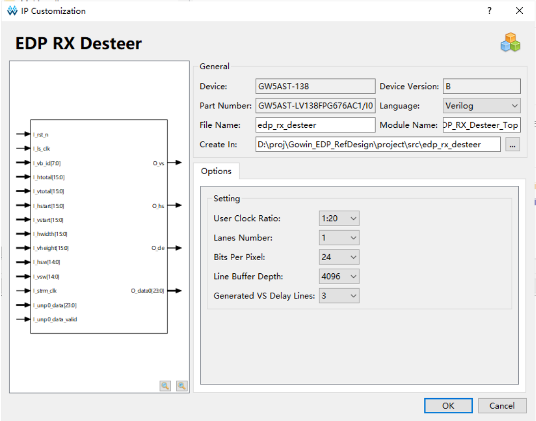
图 4-3 EDP RX Desteer IP 核接口示意图
