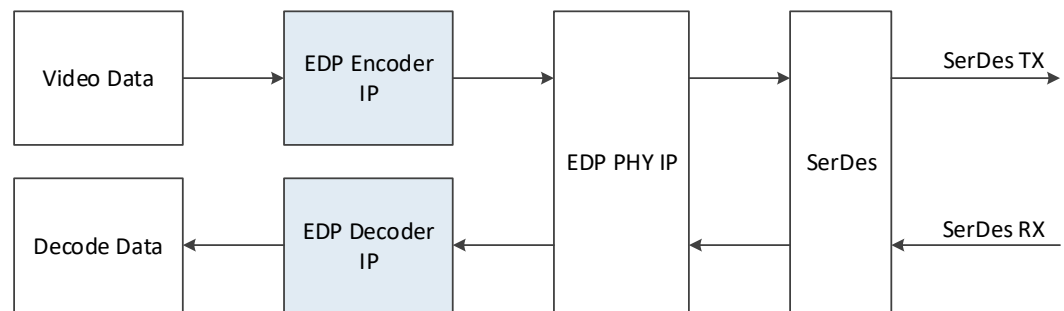
图 3-1 系统框图
