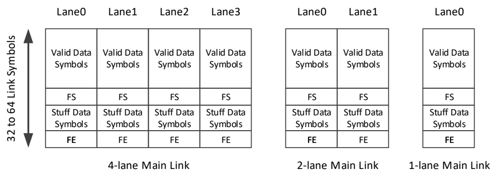
图 3-6 Transfer Unit 示意图
