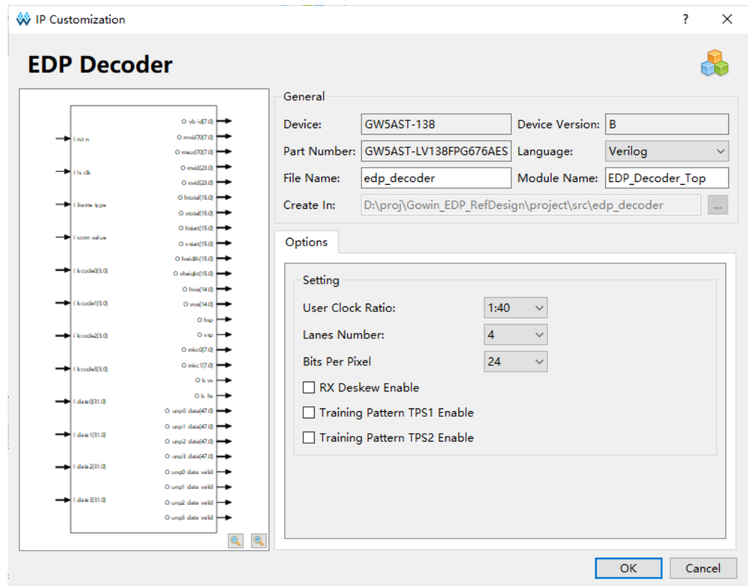
图 4-8 EDP Decoder IP 核接口示意图
