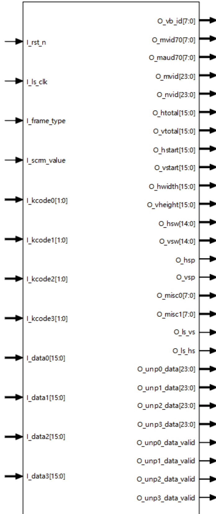
图 3-12 EDP Decoder IO 端口示意图
