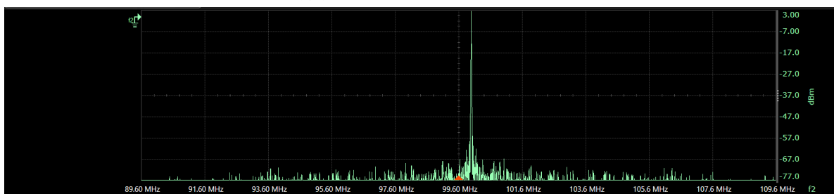
图 6-2 100MHz 时钟的频域
