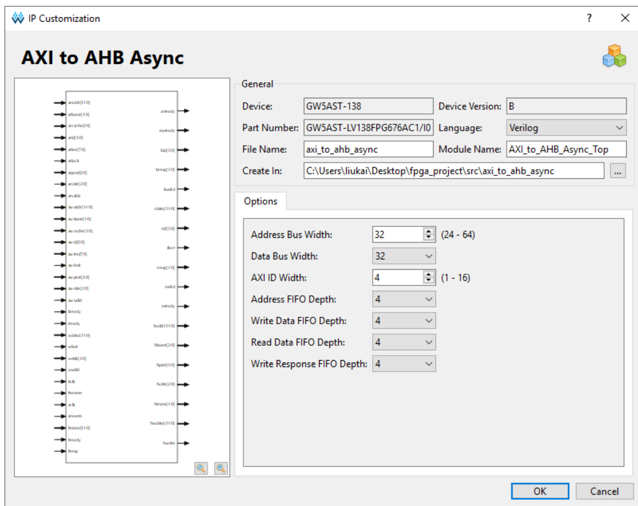
图 6-1 界面配置
