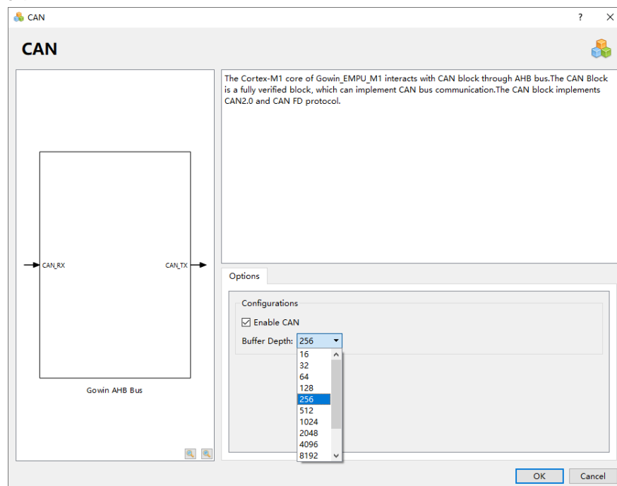
图 3-12 CAN 配置
