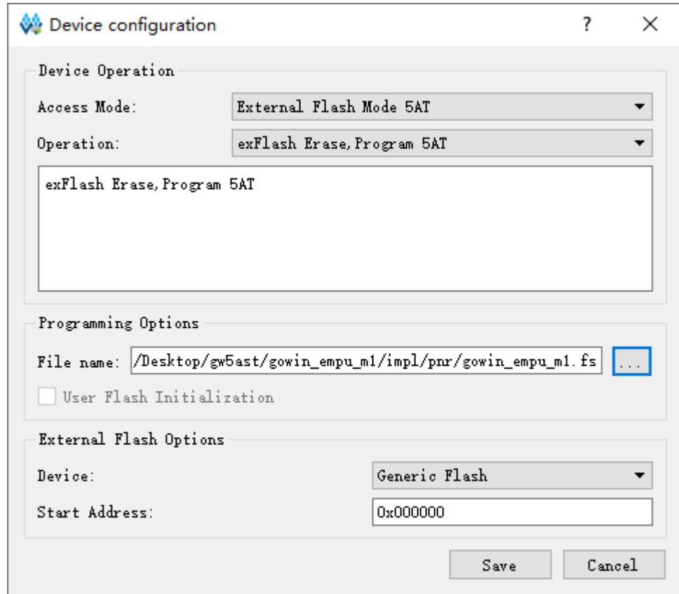
图 3-37 Arora V External Flash Mode 配置
