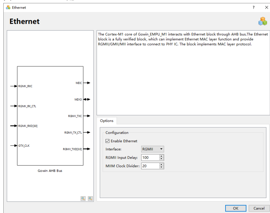
图 3-13 Ethernet 配置
