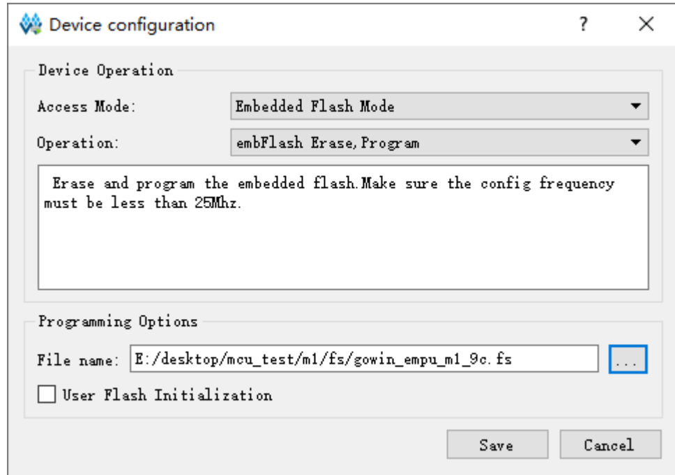
图 3-34 小蜜蜂 LittleBee 家族 Embedded Flash Mode 配置
