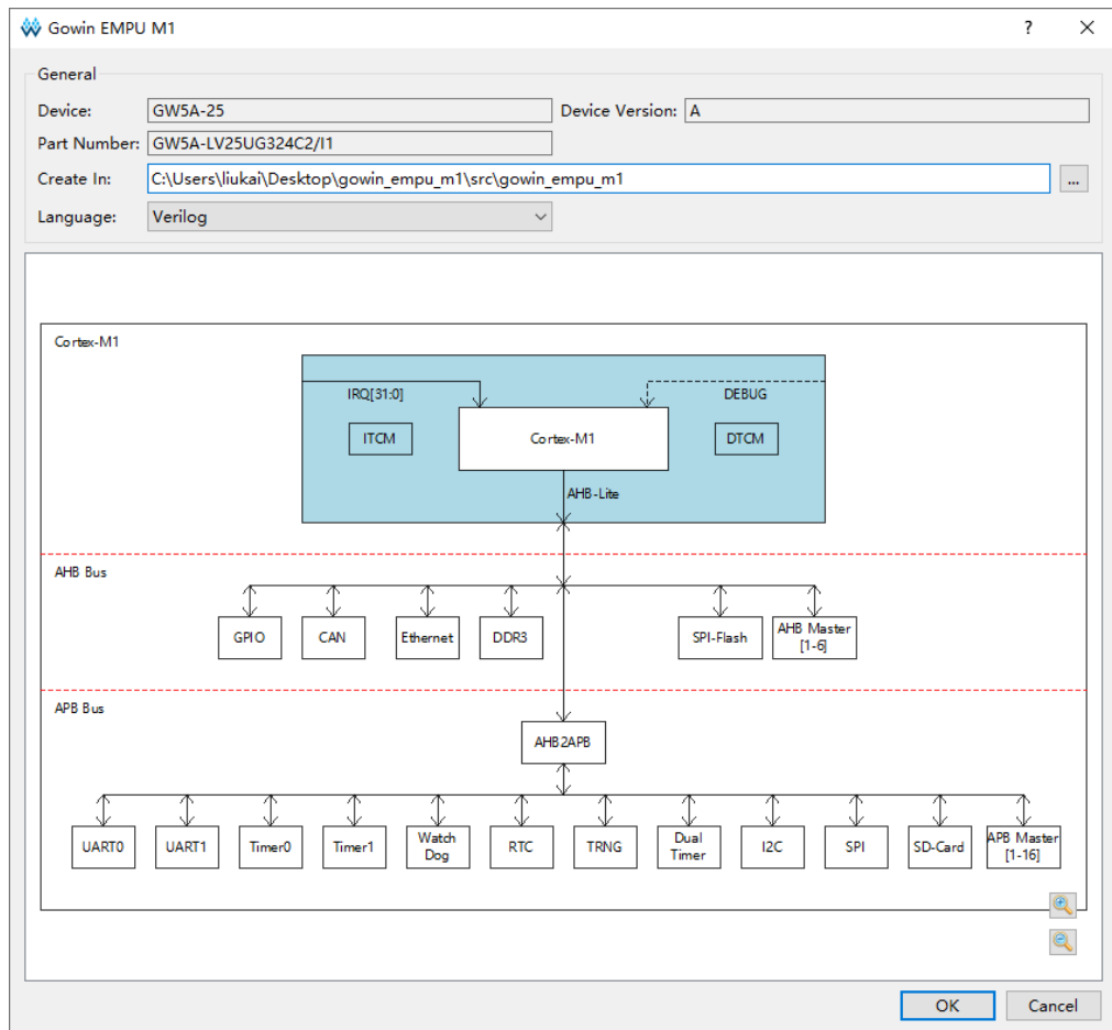
图 3-6 系统配置
