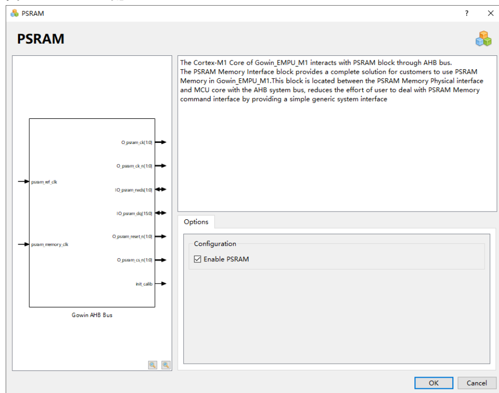
图 3-27 PSRAM 配置
