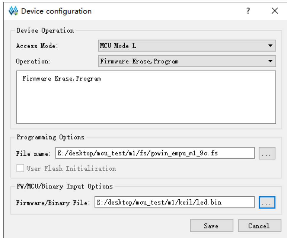
图 3-35 小蜜蜂 LittleBee 家族 MCU Mode 配置
