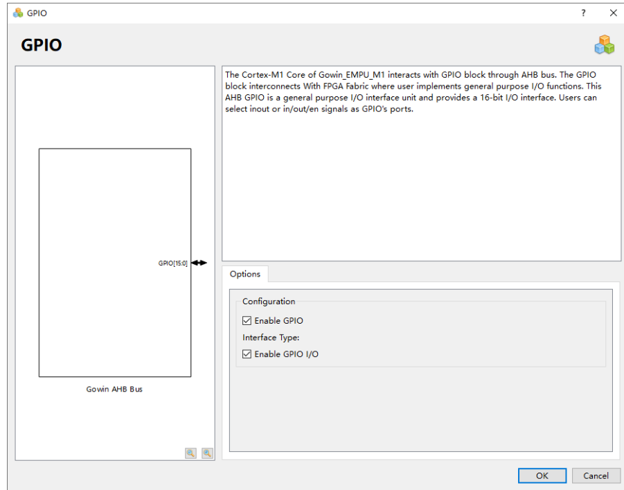
图 3-11 GPIO 配置
