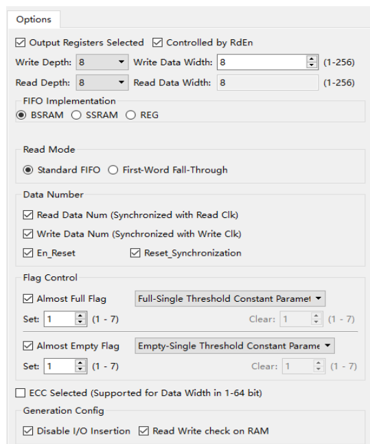
图 4-5 FIFO HS 配置
