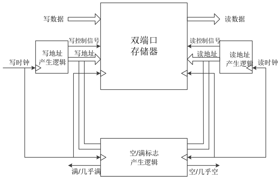
图 2-1 FIFO HS IP 结构示意图
