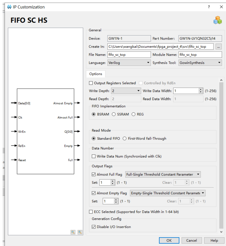
图 5-1 FIFO SC HS IP 配置页面
