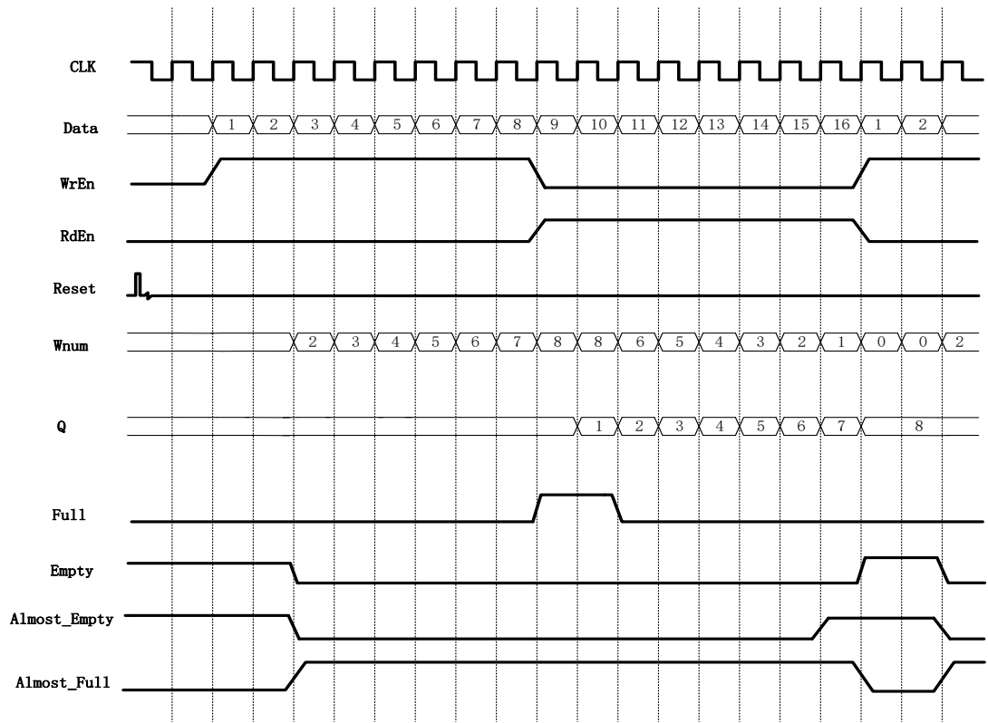
图 4-24 FIFO SC HS IP 配置时序
