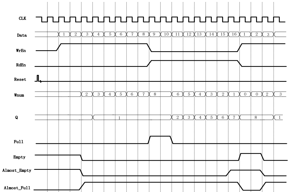
图 4-22 FIFO SC HS IP 配置时序
