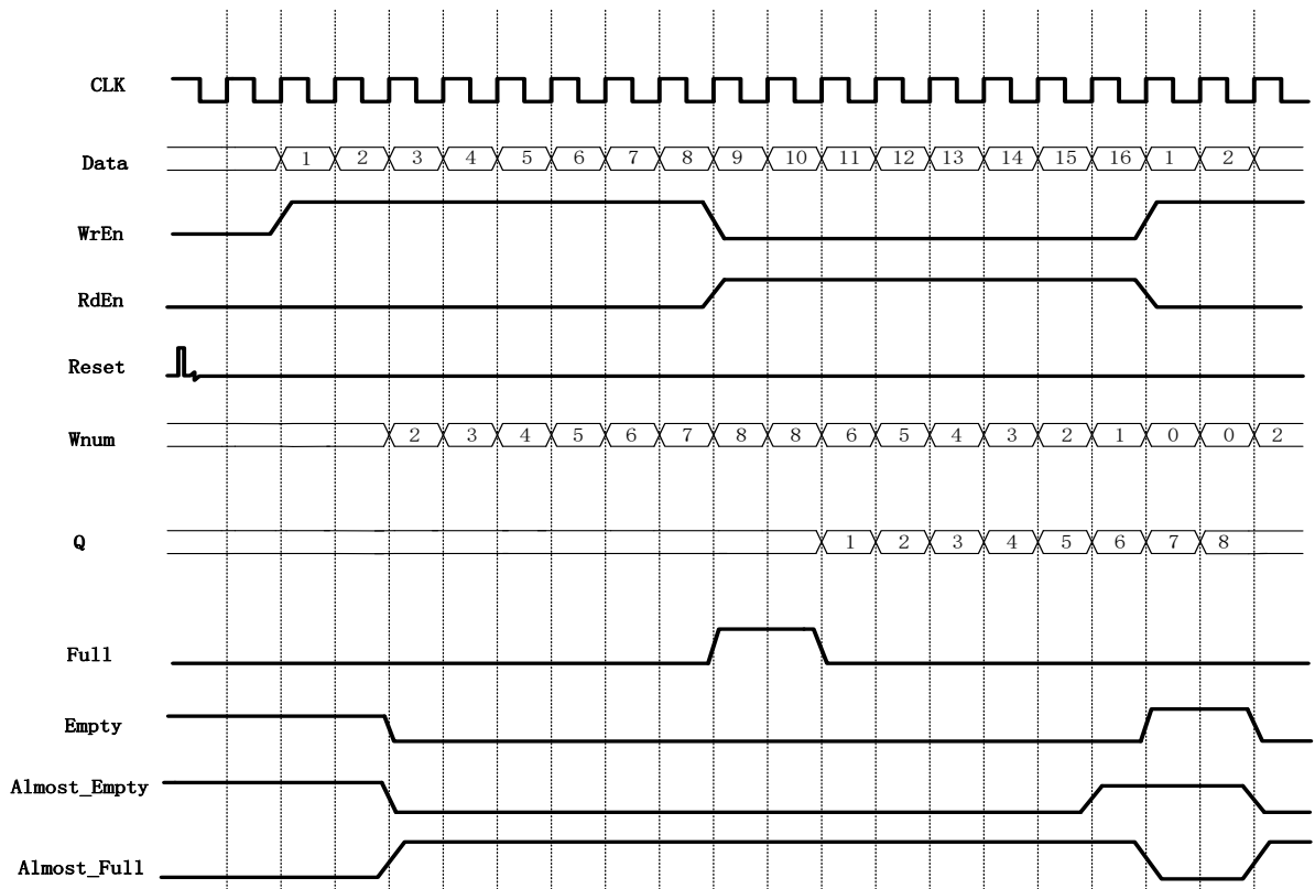
图 4-16 FIFO SC HS IP 配置时序
