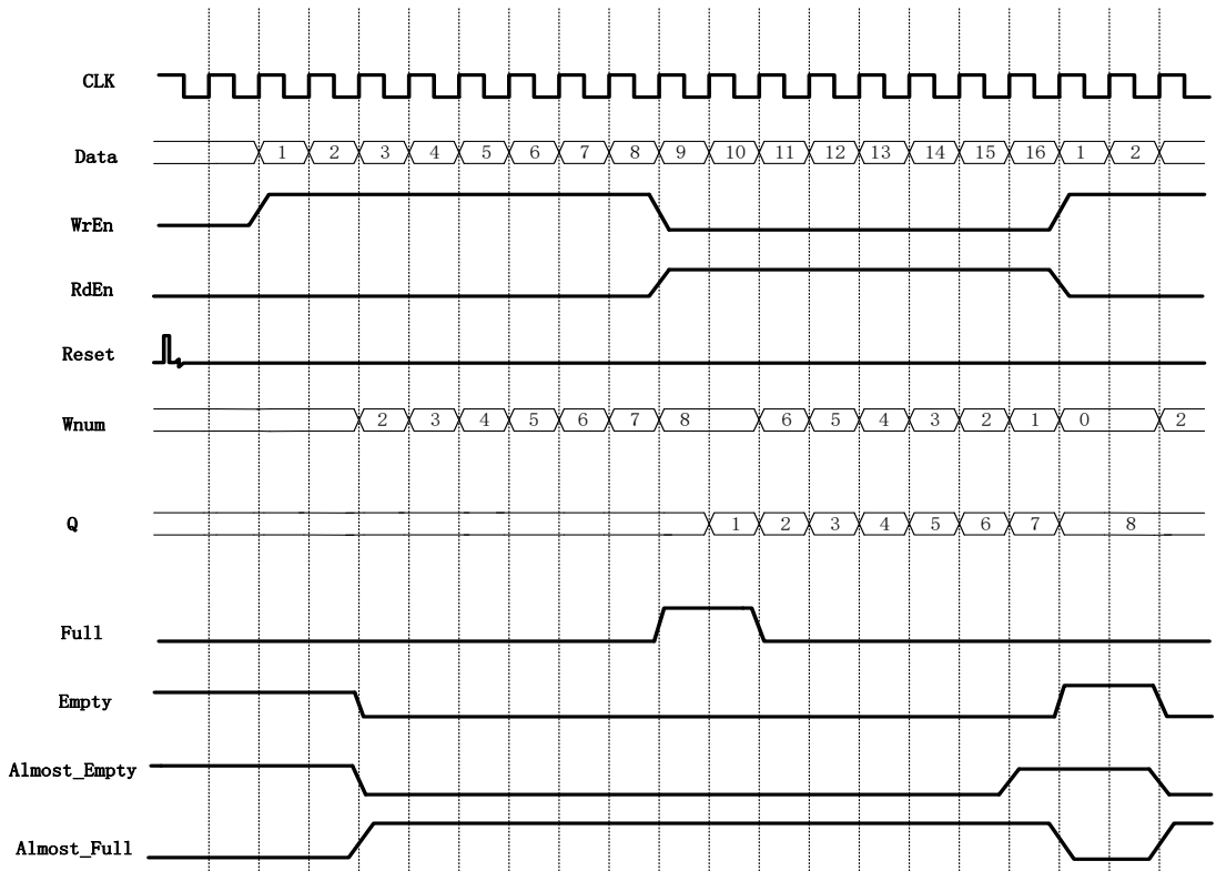
图 4-14 FIFO SC HS IP 配置时序
