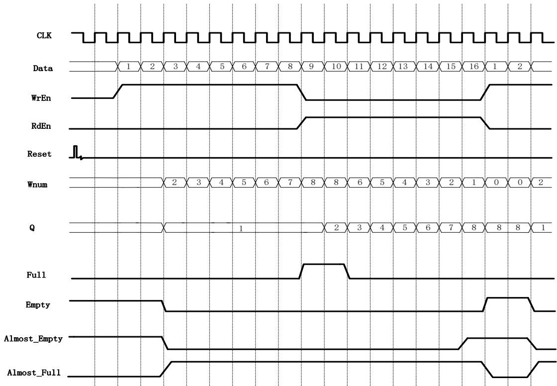
图 4-20 FIFO SC HS IP 配置时序
