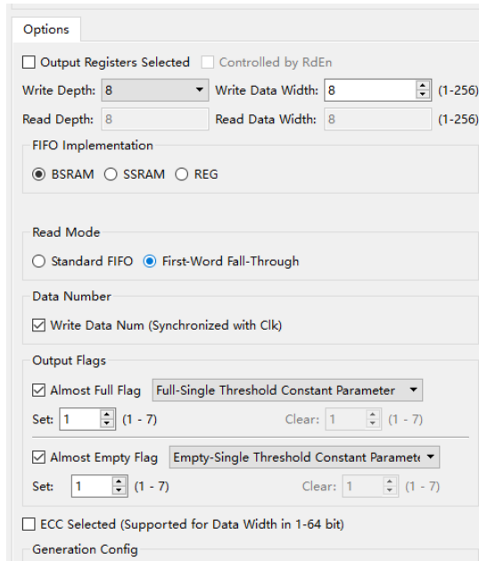
图 4-19 FIFO SC HS 配置
