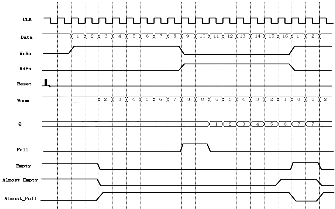
图 4-18 FIFO SC HS IP 配置时序
