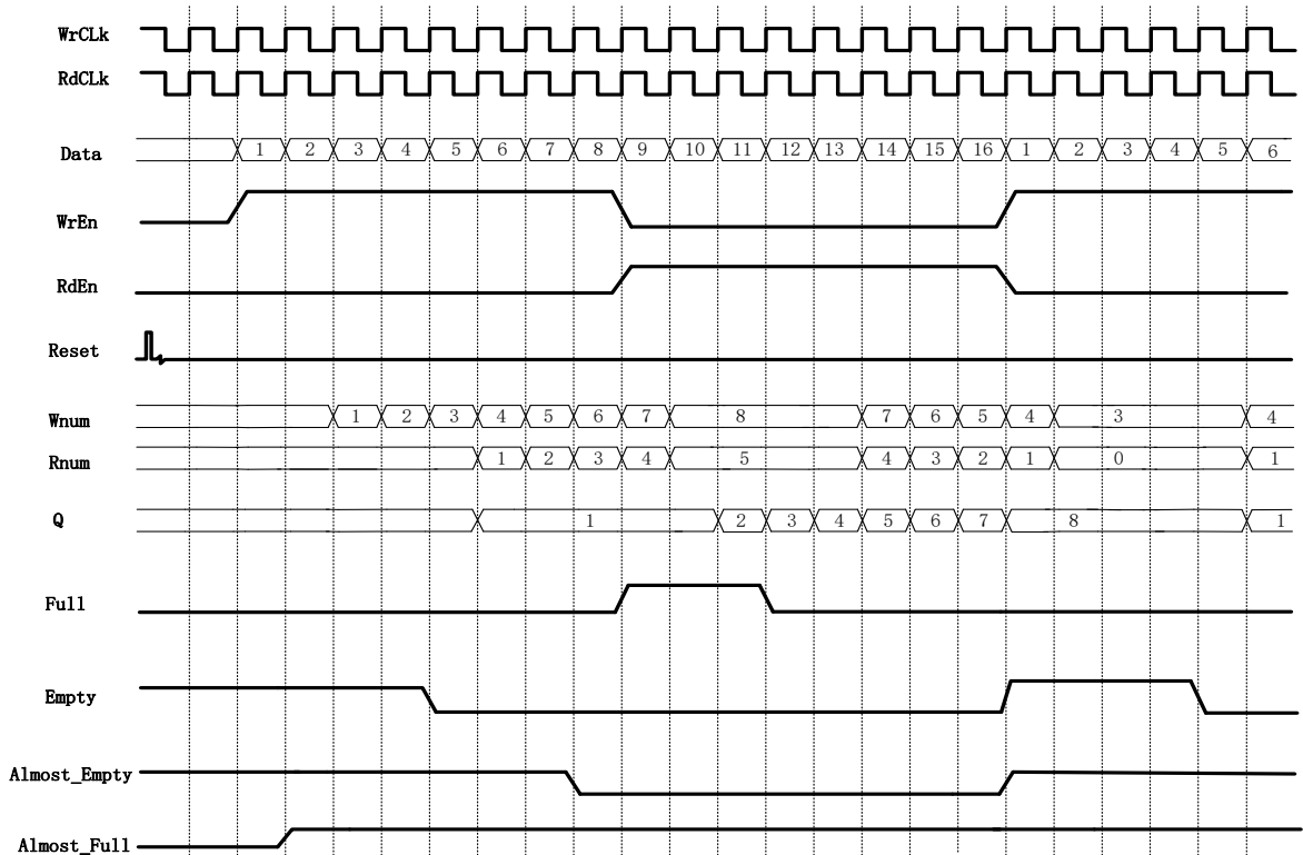
图 4-10 FIFO HS IP 配置时序
