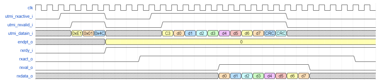
图 3-3 USB Device Controller 数据接收时序图
