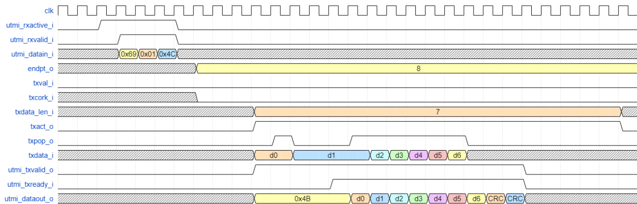
图 3-7USB Device Controller 控制端点数据发送时序
