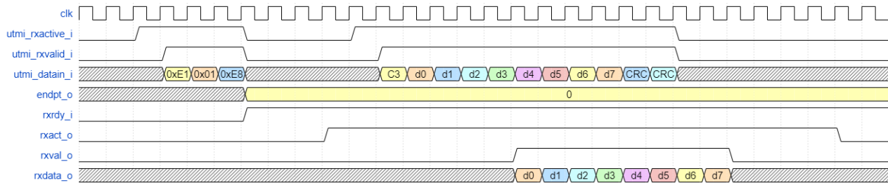
图 3-6USB Device Controller 控制端点数据接收时序图
