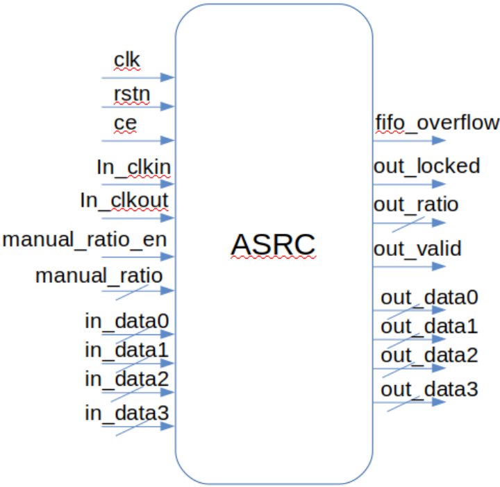
图 4-2 Gowin ASRC IP 端口图
