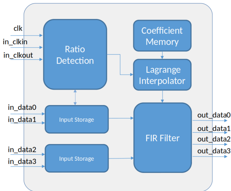
图 4-1 Gowin ASRC IP 实现框图
