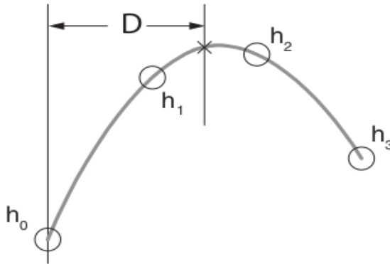
图 2-3 阶拉格朗日插值对滤波器系数处理示意图
