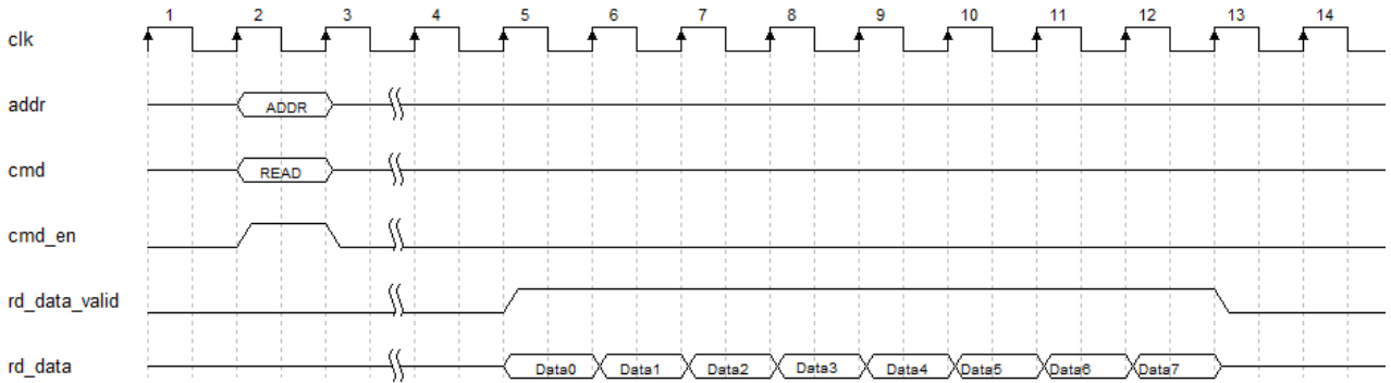
图 4-12 突发长度为 32 时读数据时序图
