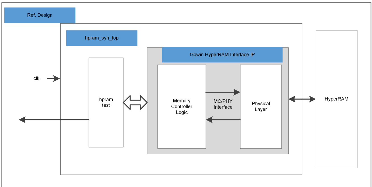
图 7-1 参考设计基本结构框图
