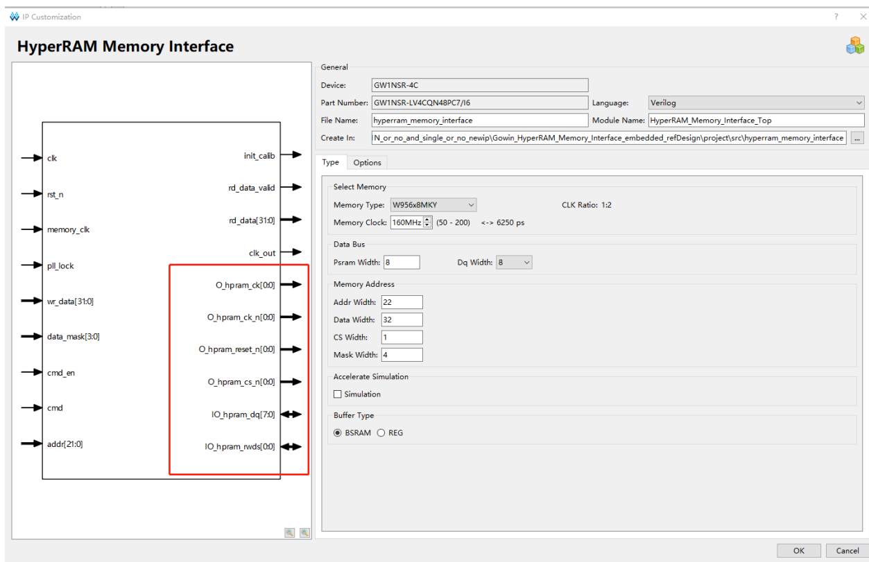
图 8-3 IP 核接口示意图
