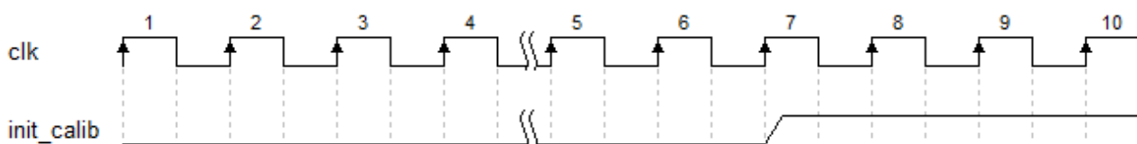
图 4-4 初始化完成信号时序图
