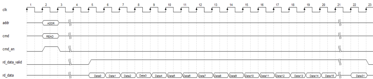
图 4-14 突发长度为 128 时读数据时序图
