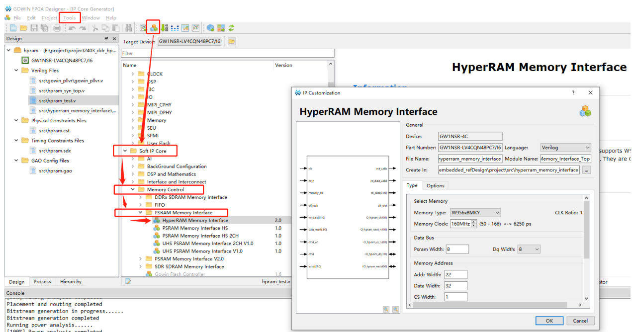
图 8-2 打开 HyperRAM Memory Interface IP 核
