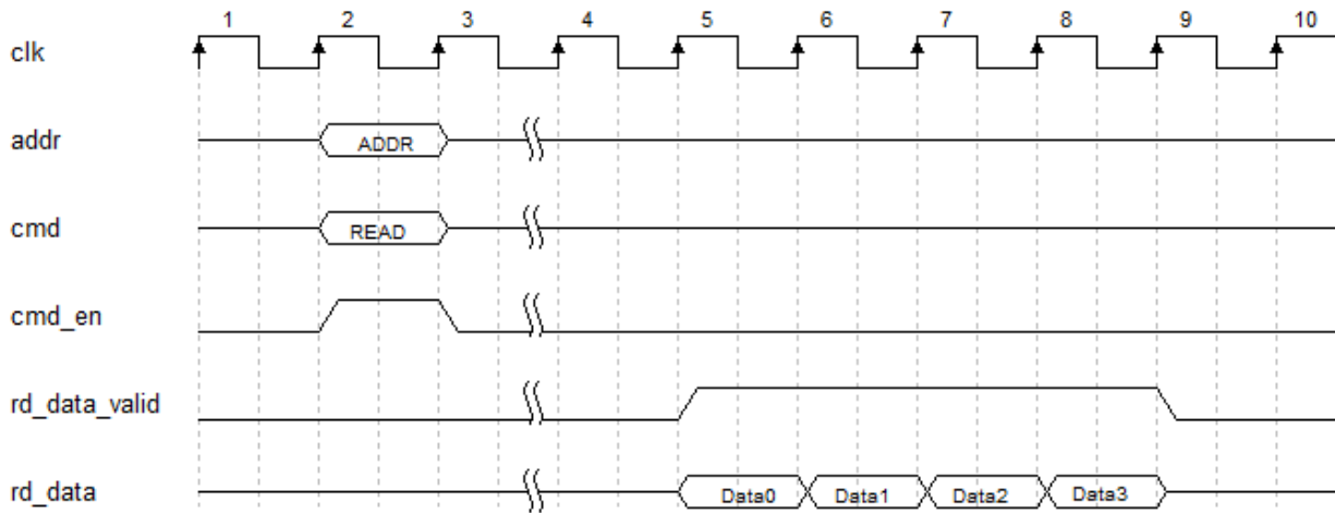
图 4-11 读数据端口时序图
