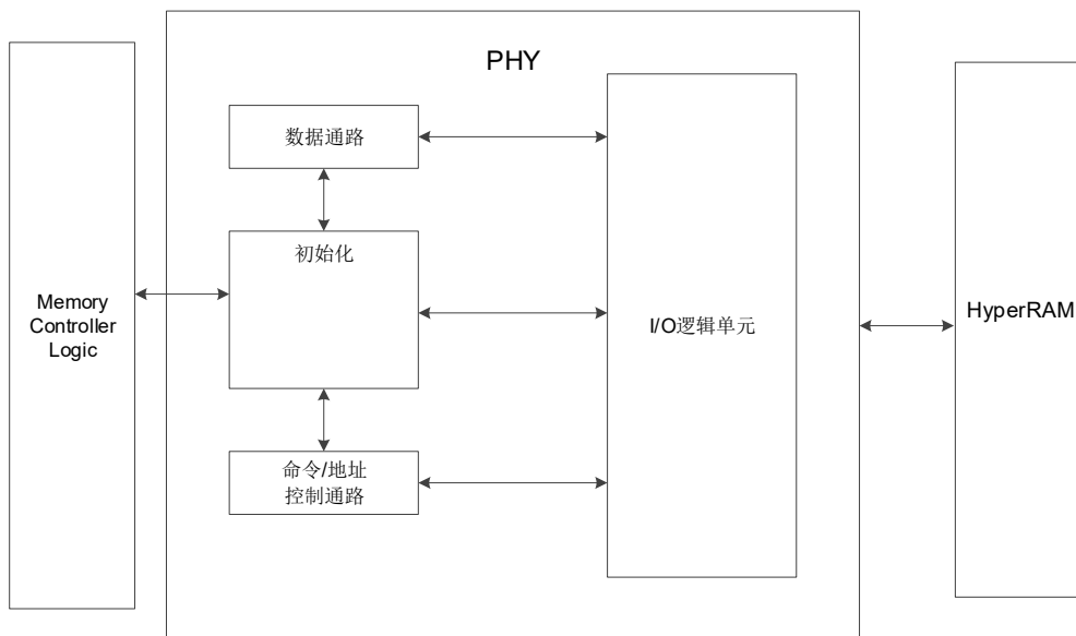
图 4-3 HyperRAM PHY 基本结构图
