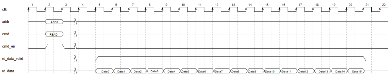
图 4-13 突发长度为 64 时读数据时序图
