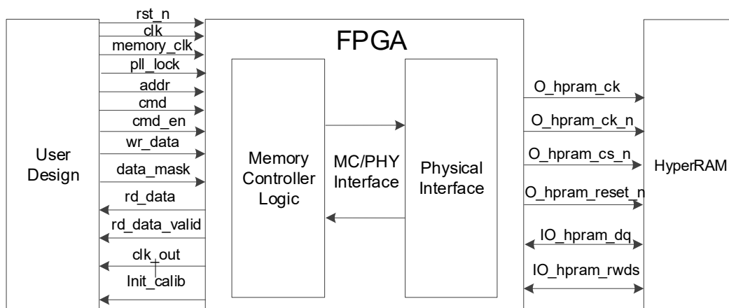
图 4-1 Gowin HyperRAM Memory Interface IP 结构图
