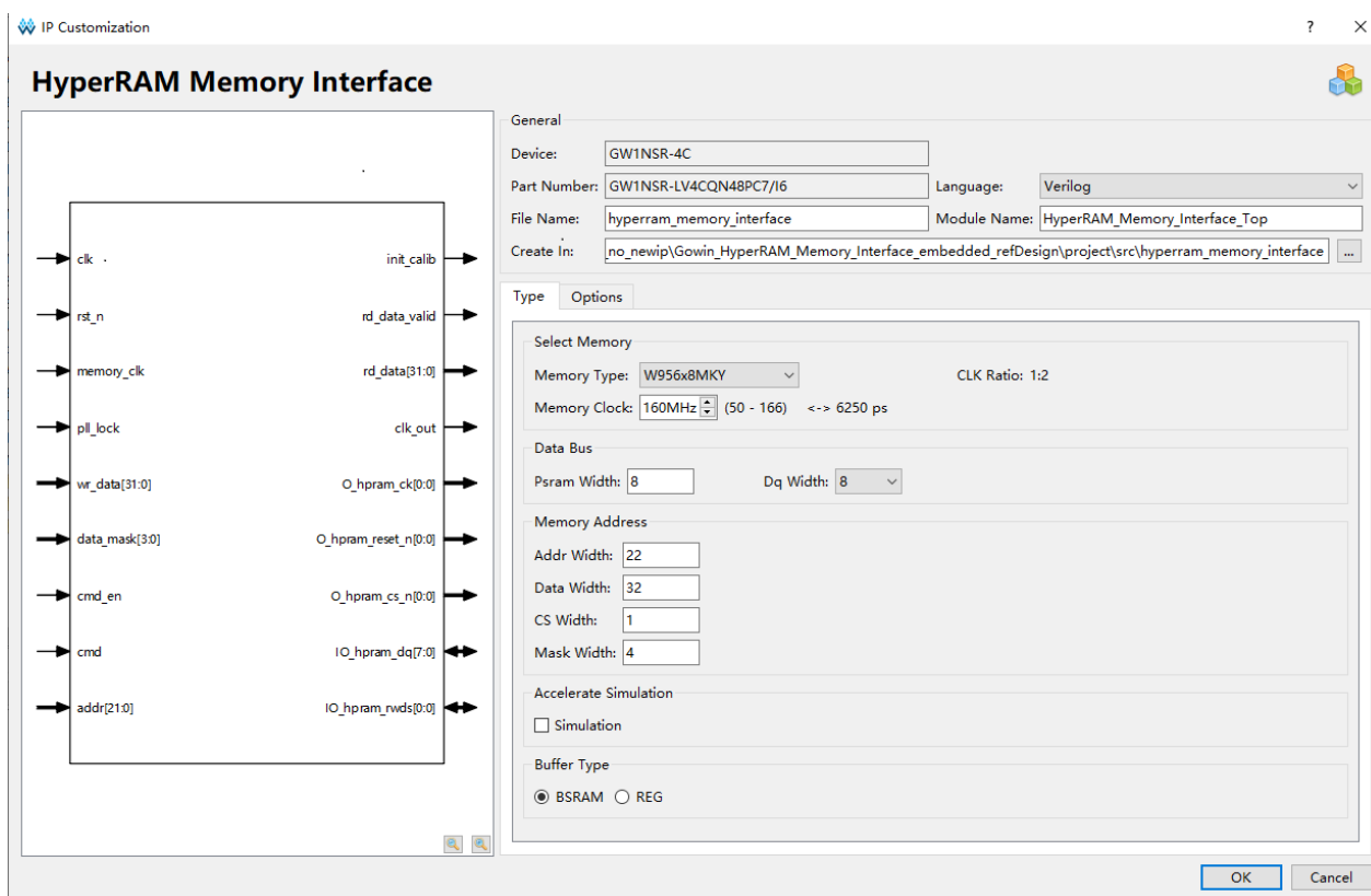
图 8-5 Type 选项卡
