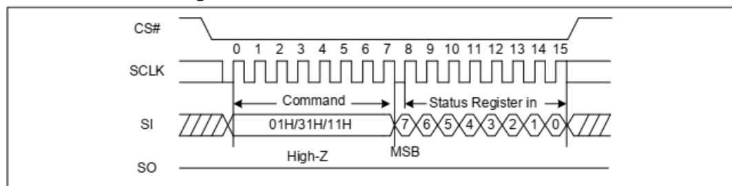
图 3-6 Write Status Register 时序图
