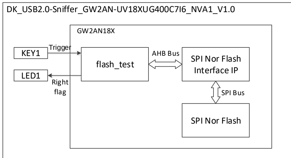
图 5-2 参考设计实例二基本结构图
