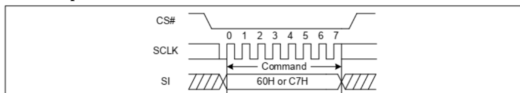
图 3-12 Chip Erase 时序图
