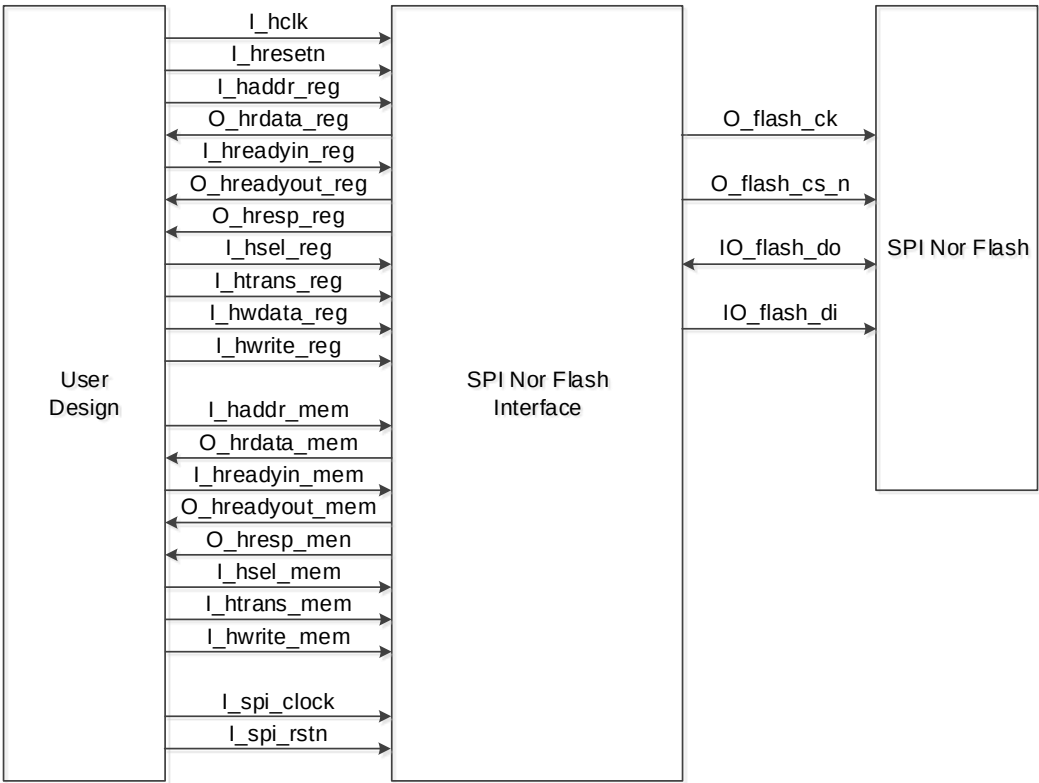
图 3-1 系统框图
