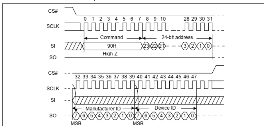
图 3-13 Read Manufacture ID/Device ID 时序图
