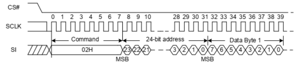
图 3-17 SPI Flash 写接口时序图
