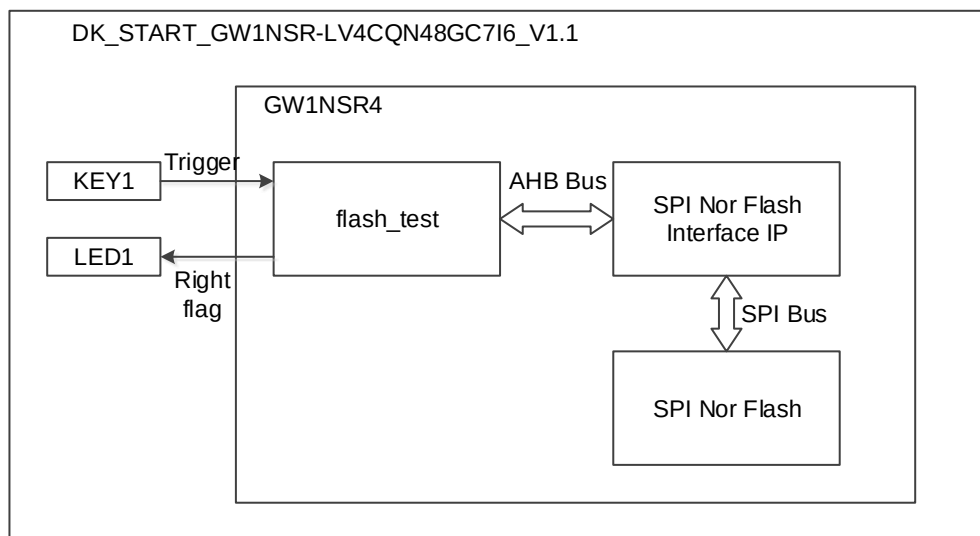
图 5-1 参考设计实例一基本结构图
