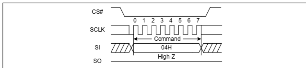
图 3-4 Write Disable 时序图
