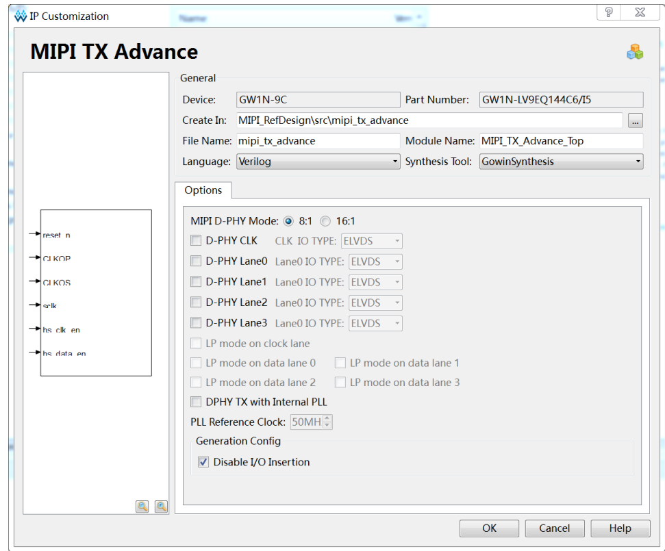
图 7-2 MIPI D-PHY TX Advance 配置页面
