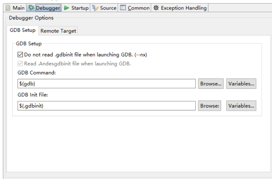
图 4-60 Debugger 选项卡
