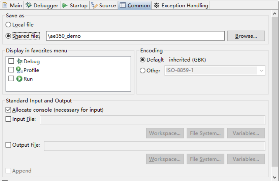
图 4-63 Common 选项卡
