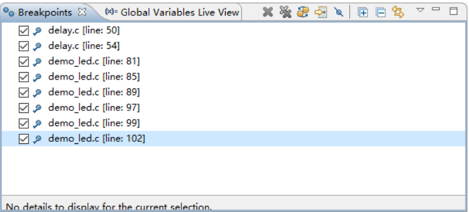
图 4-53 断点视图
