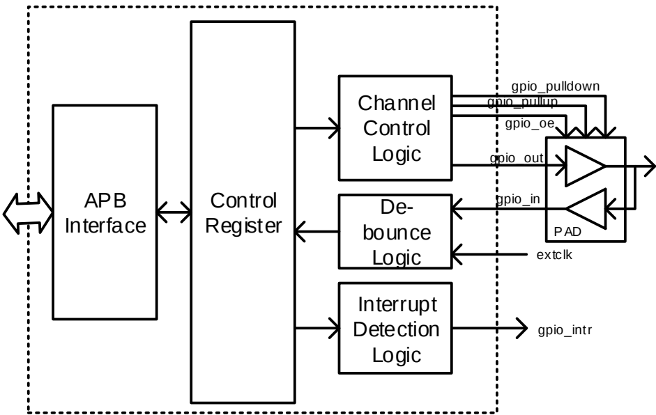
图 8-1 GPIO 结构框图
