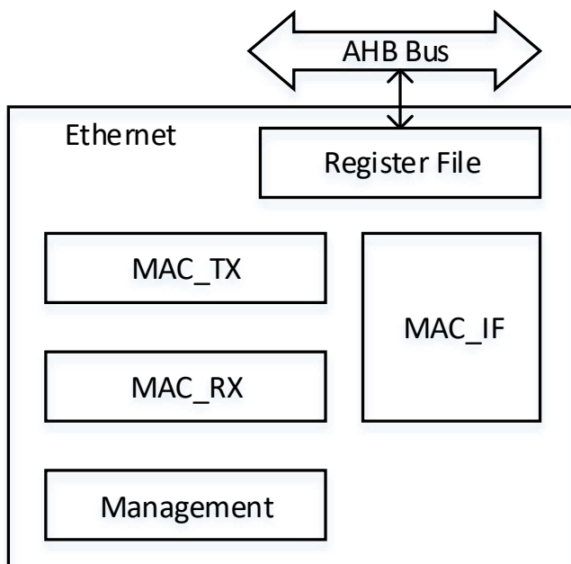
图 18-1 Ethernet 结构框图
