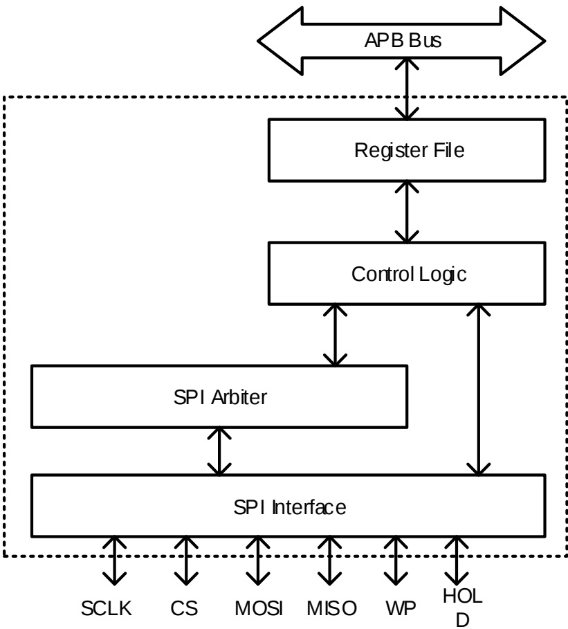
图 10-1 SPI 结构框图
