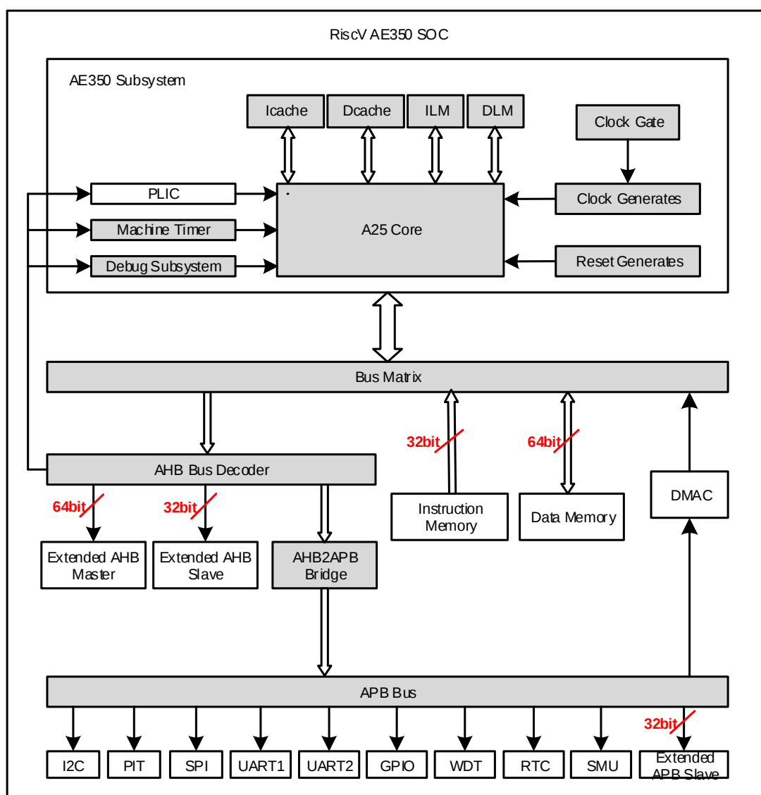
图 2-1 系统架构
