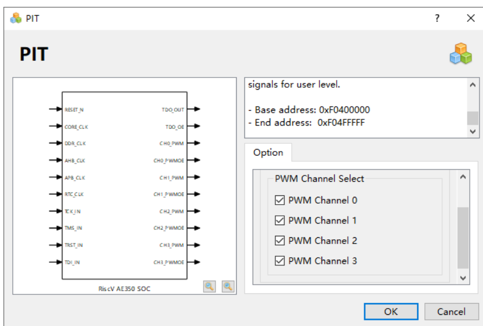
图 8-11 PIT 配置
