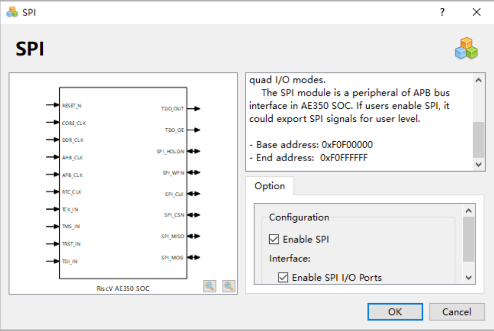
图 8-12 SPI 配置
