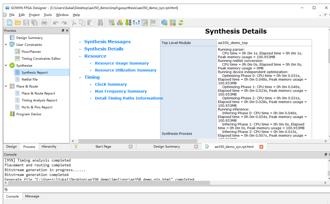
图 8-28 综合
