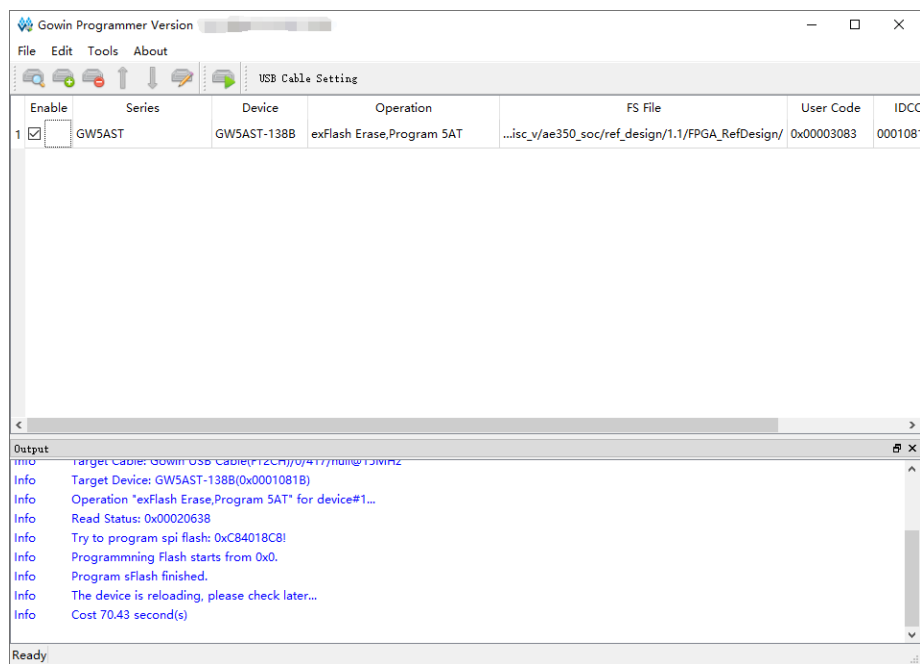
图 8-31 下载码流文件
