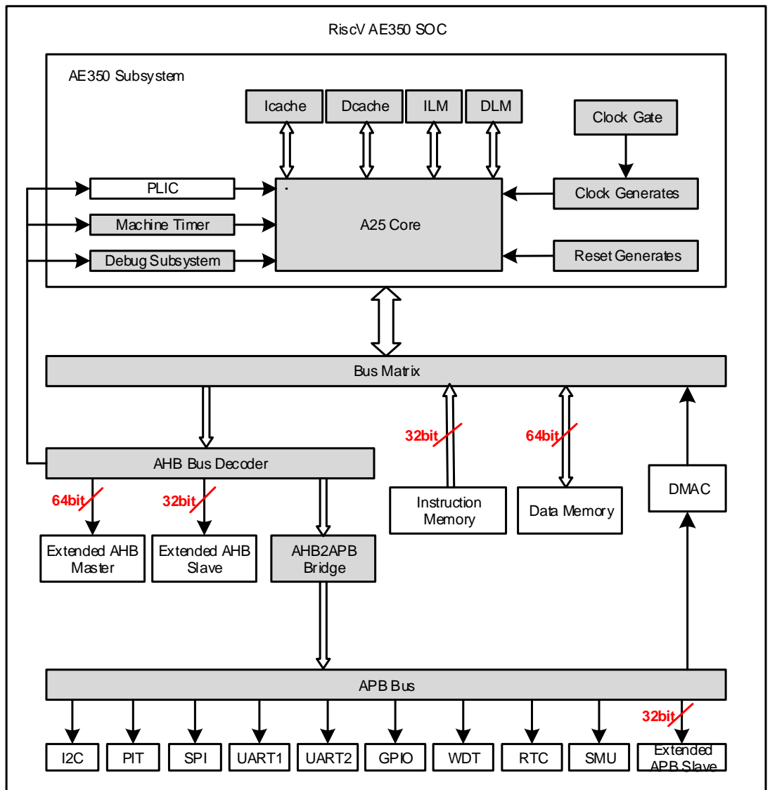
图 2-1 系统架构
