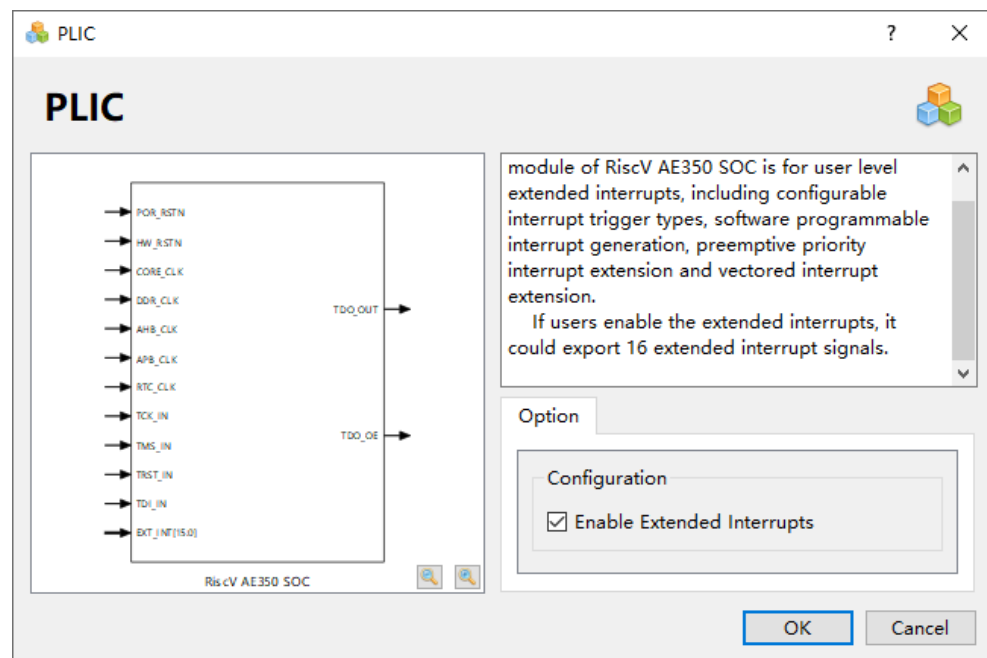
图 8-7 PLIC 配置
