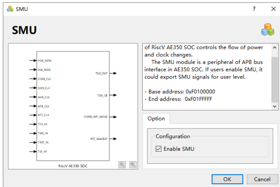
图 8-17 SMU 配置
