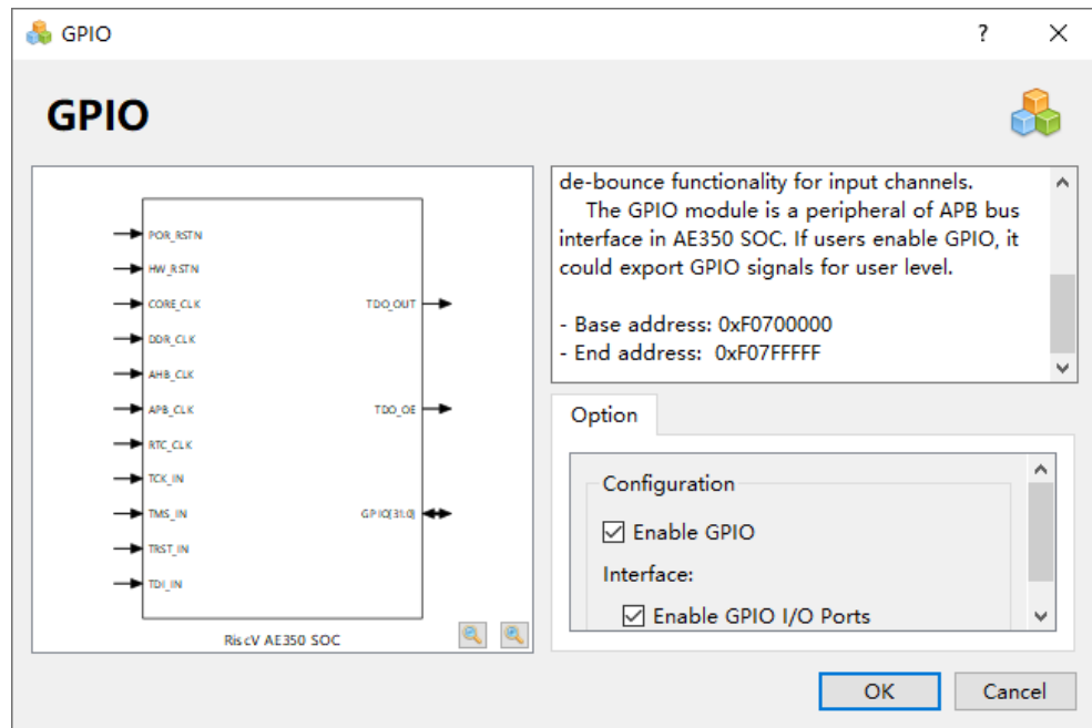
图 8-14 GPIO 配置
