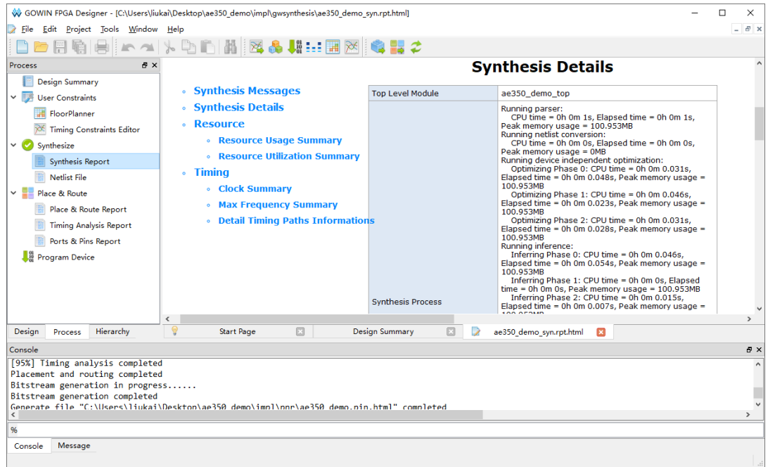
图 8-28 综合
