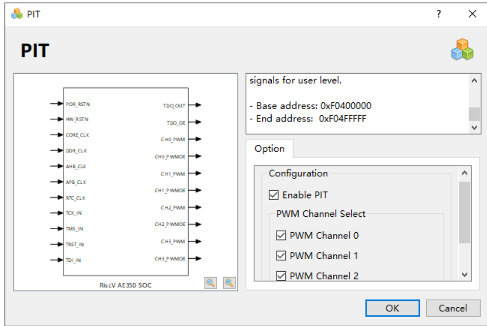
图 8-11 PIT 配置
