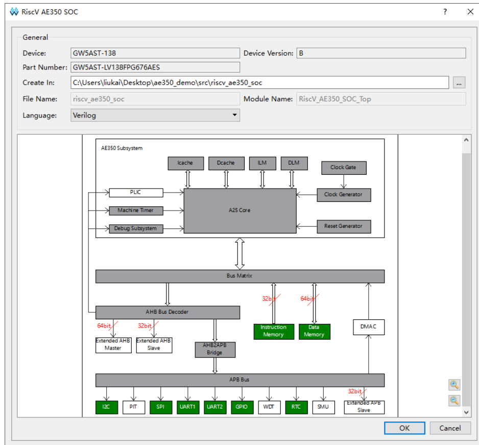
图 8-22 RiscV_AE350_SOC IP 设计
