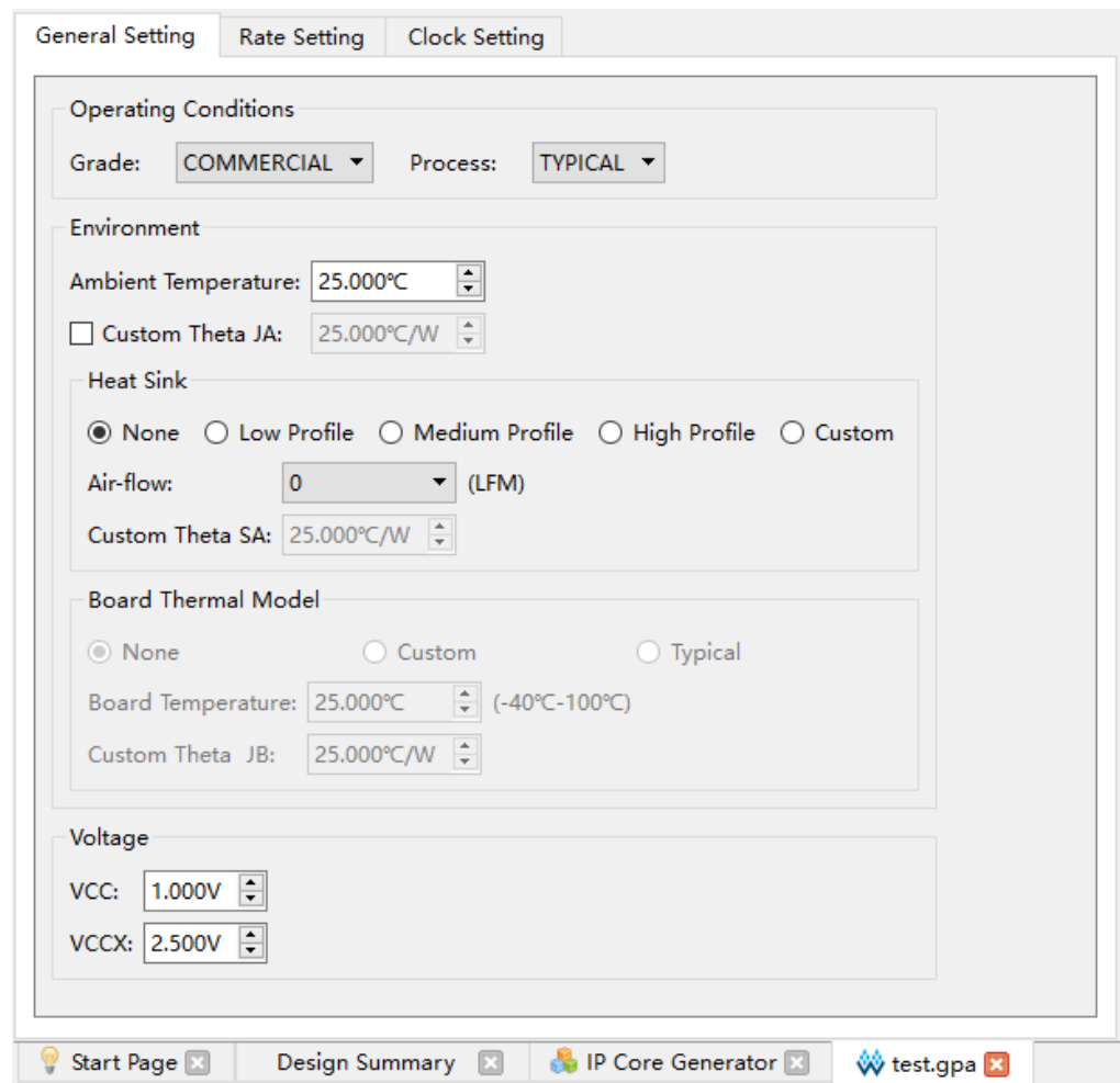
图 5-7 GPA 配置文件窗口
