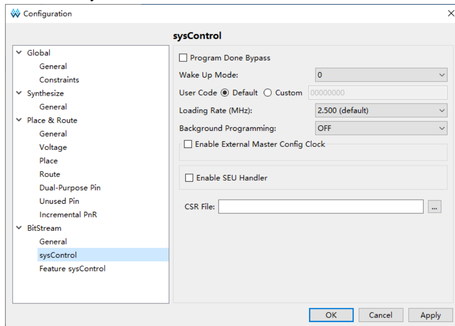
图 4-29 配置 sysControl 选项
