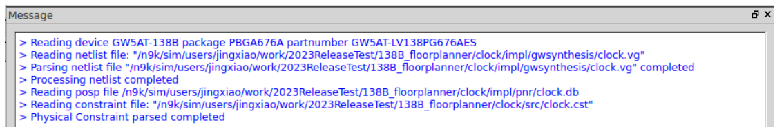
图 3-51 Message 窗口
