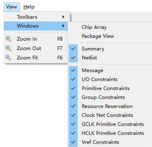
图 3-24 Windows 菜单
