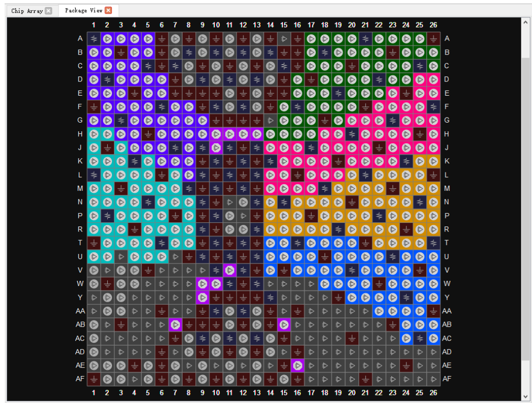
图 3-30 GW5AT-138-FPBGA676A Package view 窗口
