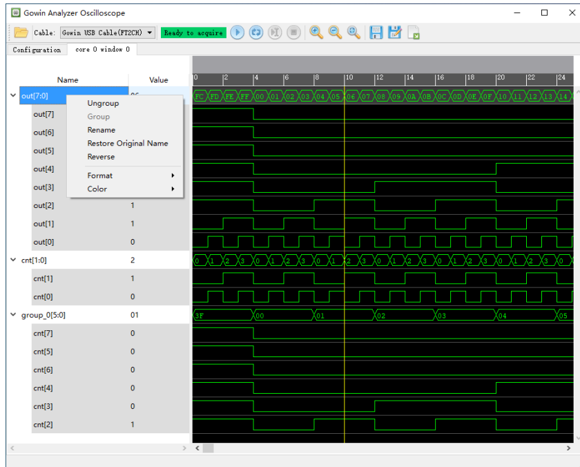
图 4-11 单个信号右键菜单（Standard Mode）
