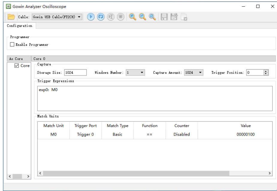
图 4-13 Reload GAO 配置文件
