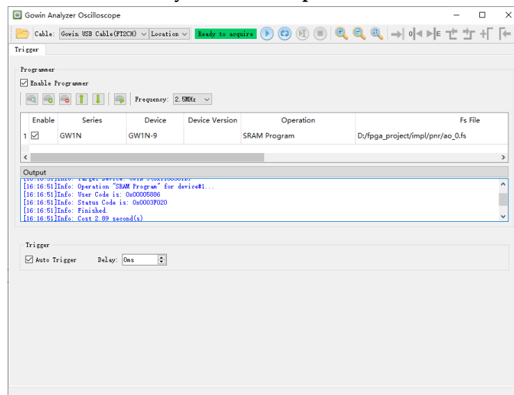
图 4-22 Gowin Analyzer Oscilloscope 工具窗口（Lite Mode）
