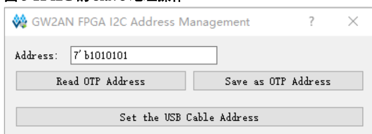
图 3-11 I2C 的 slave 地址操作
