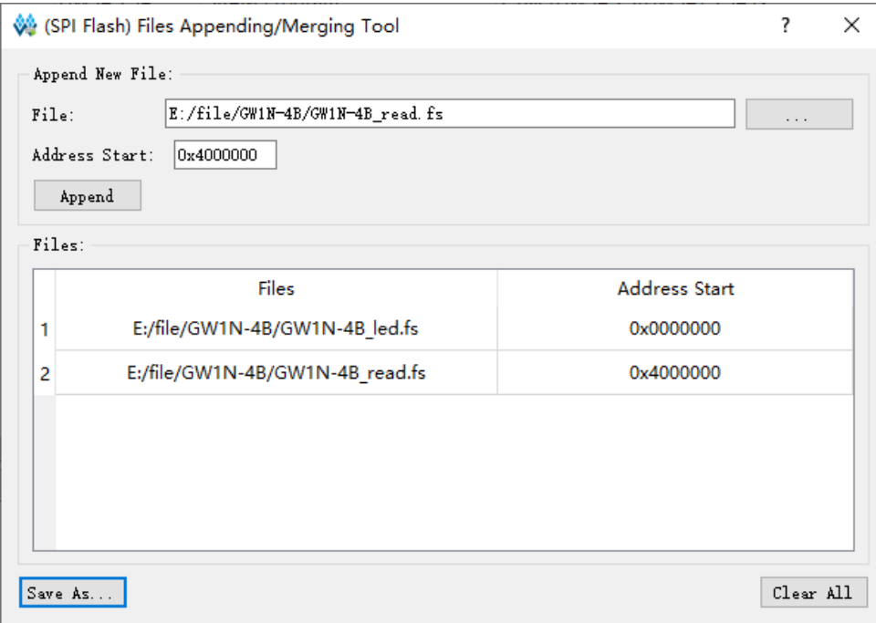
图 3-27 数据流文件合并界面
