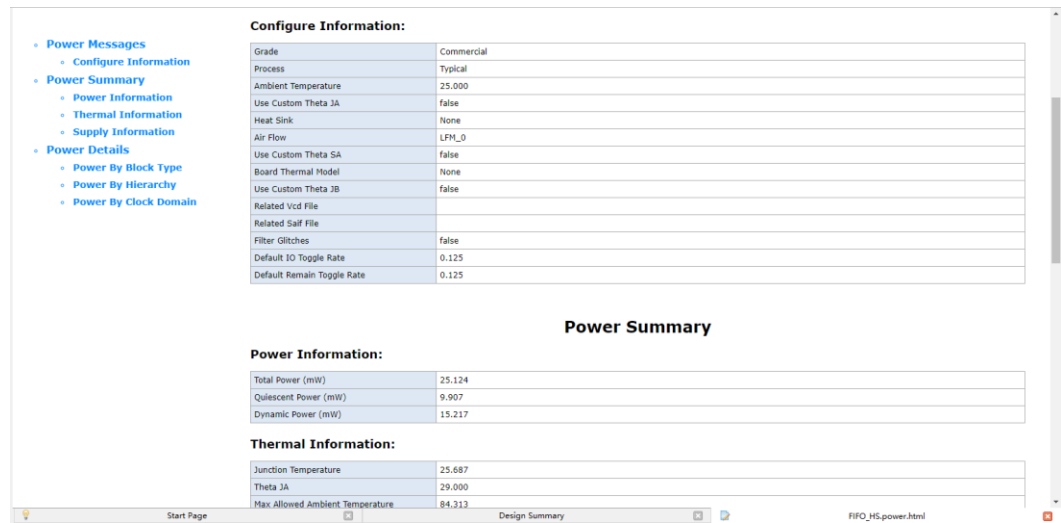
图 3-36 功耗分析报告
