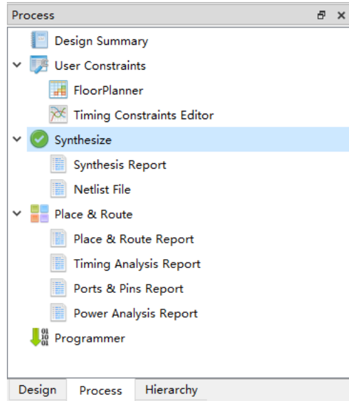
图 3-14 综合完成
