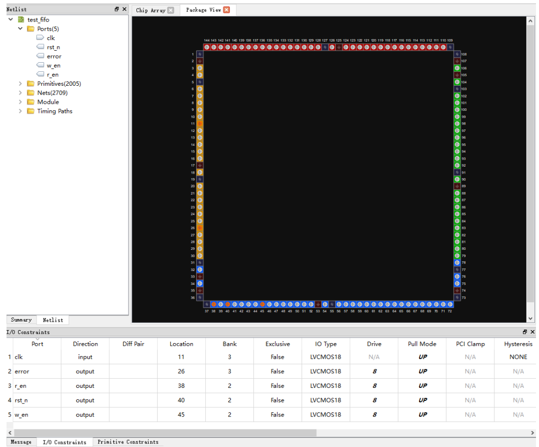
图 3-17 I/O 约束
