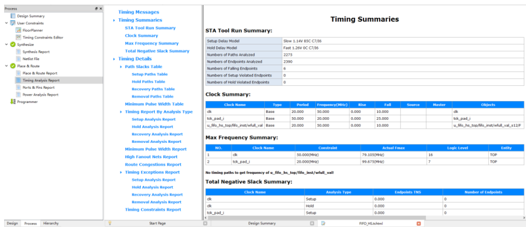
图 3-35 时序报告
