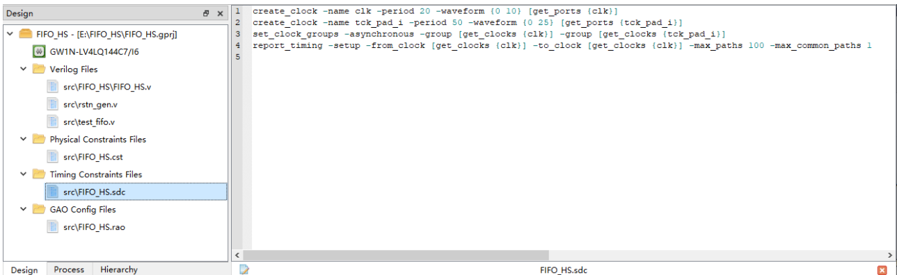
图 3-21 时序约束显示
