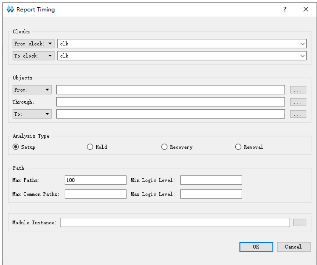
图 3-20 时序报告约束
