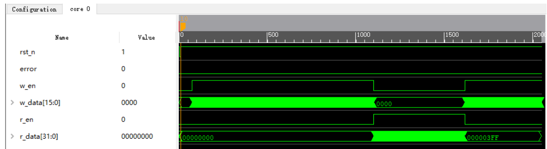
图 3-32 GAO 波形显示
