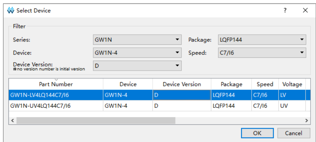
图 3-1 新建工程
