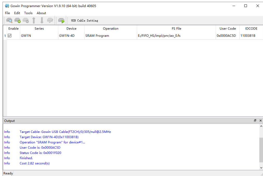
图 3-30 Programmer 界面
