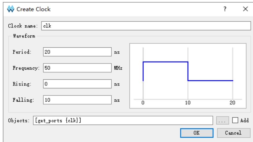
图 3-19 Clock 约束
