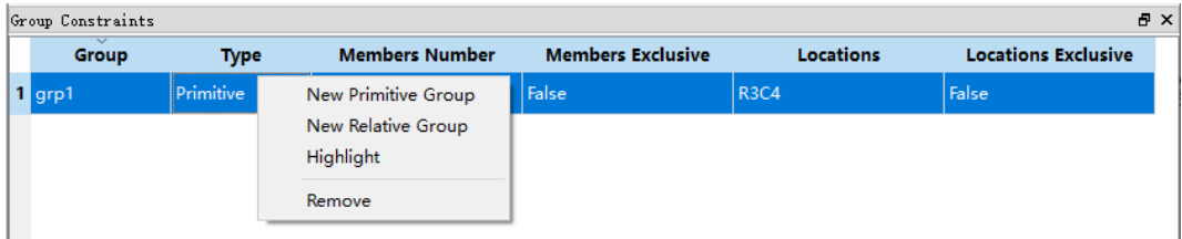
图 3-48 组约束窗口
