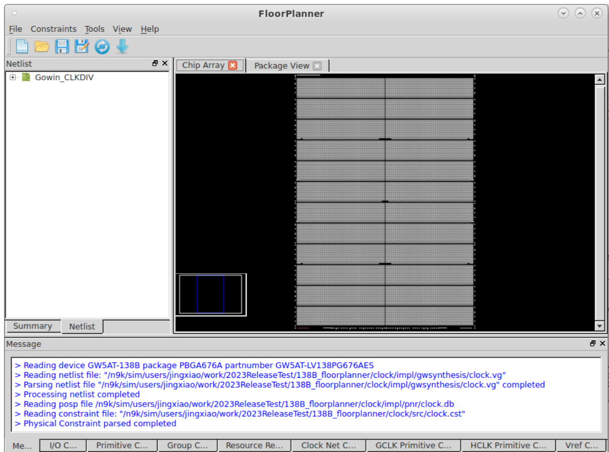
图 3-4 FloorPlanner 界面
