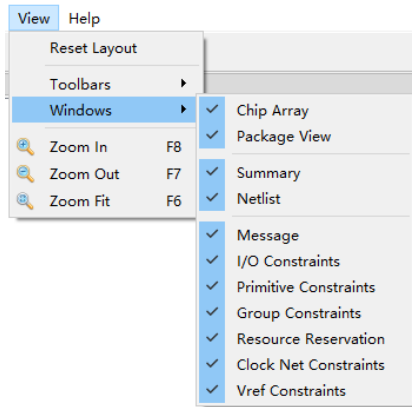
图 3-25 Windows 菜单
