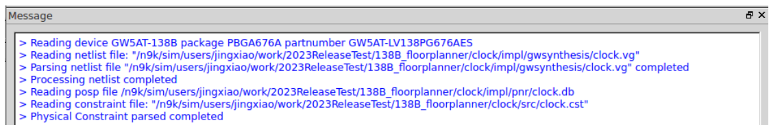
图 3-54 Message 窗口
