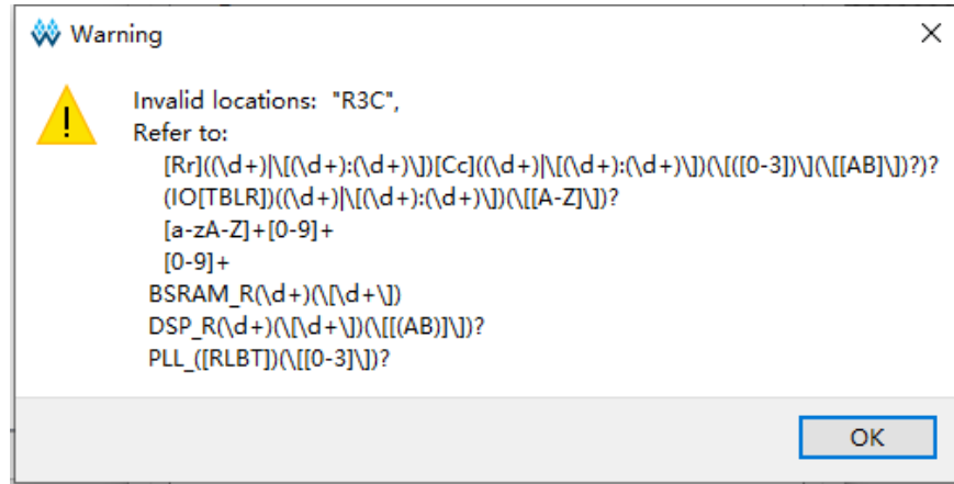
图 3-11 无效位置
