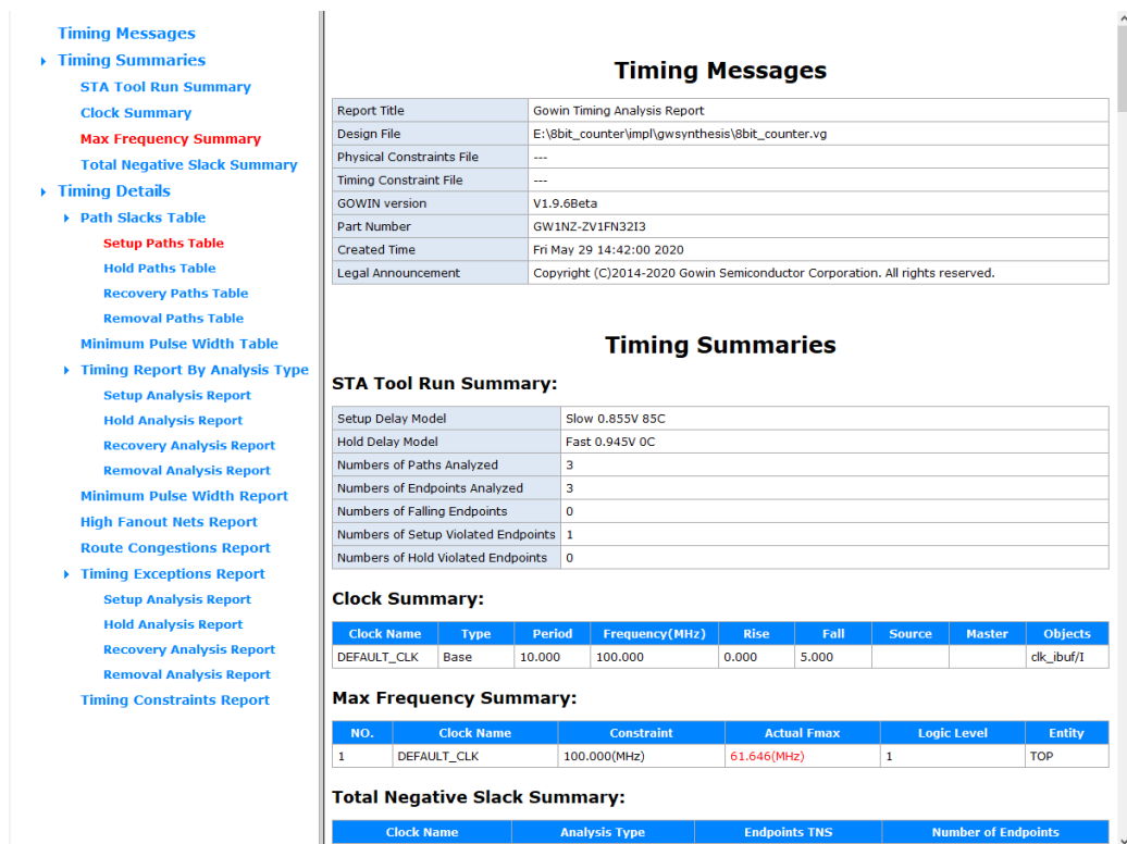
图 5-1 静态时序分析报告
