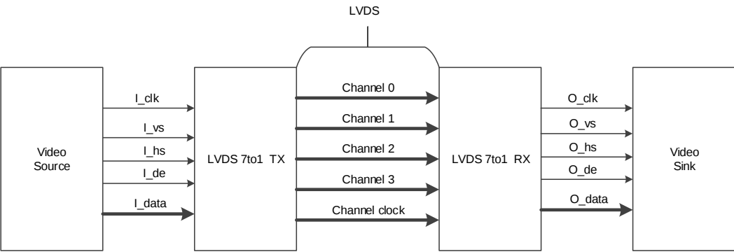
图 3-1 系统框图
