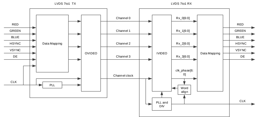
图 3-2 实现框图
