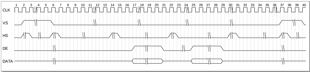
图 3-6 视频接口时序示意图
