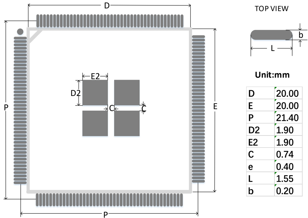
图 4-42 推荐 PCB Layout EQ176
