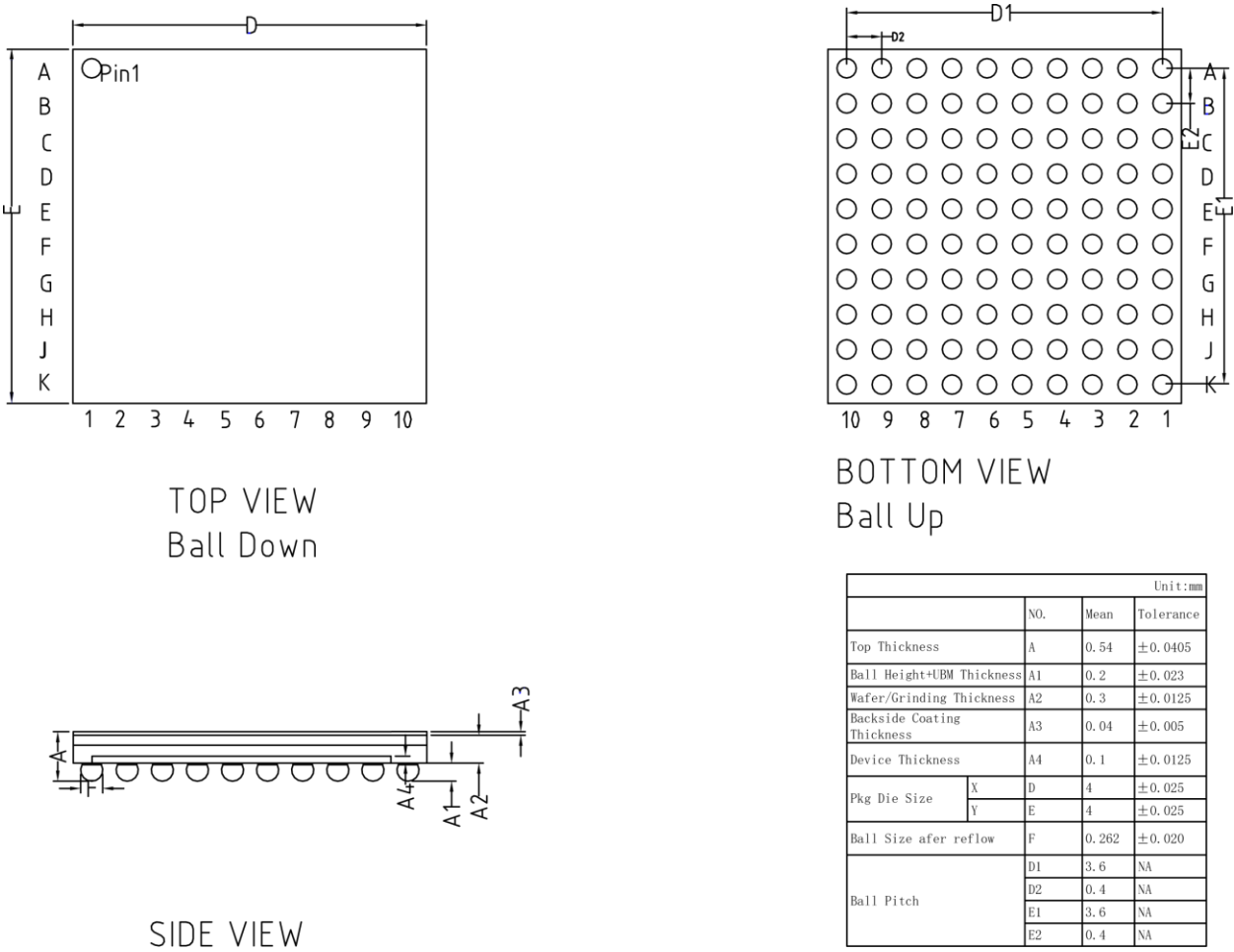
图 4-11 封装尺寸 CS100H
