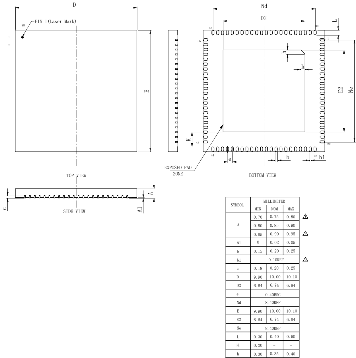
图 4-31 封装尺寸 QN88/QN88F
