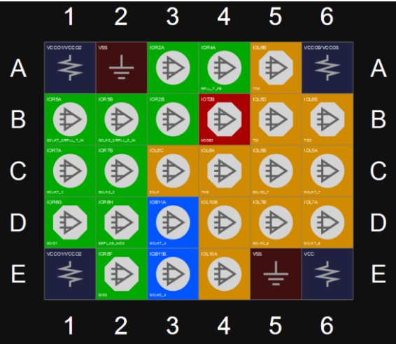
图 3-3 GW1N-1 器件 CS30 封装管脚分布示意图（顶视图）
