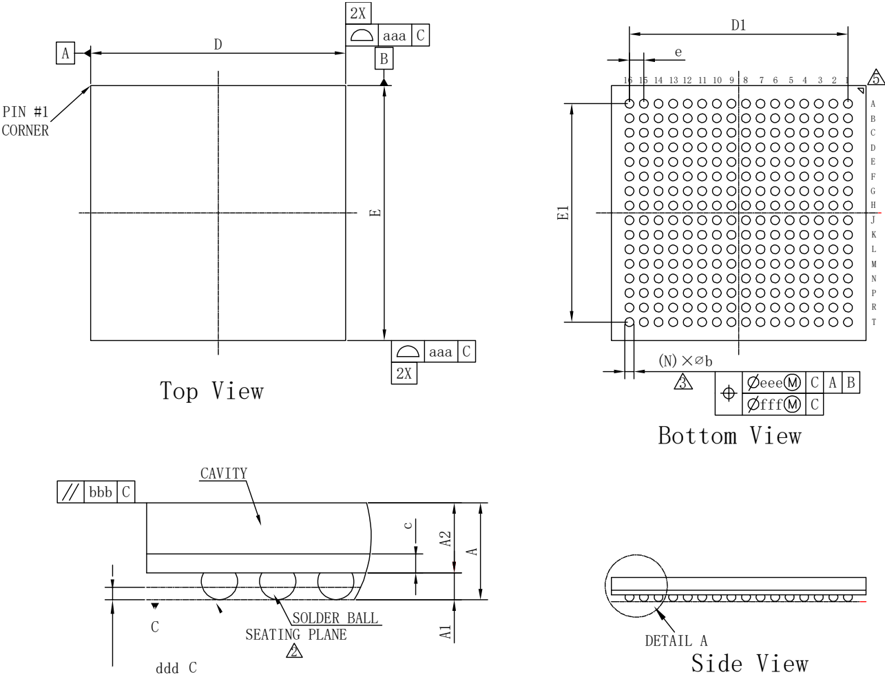
图 4-5 封装尺寸 UG256C
