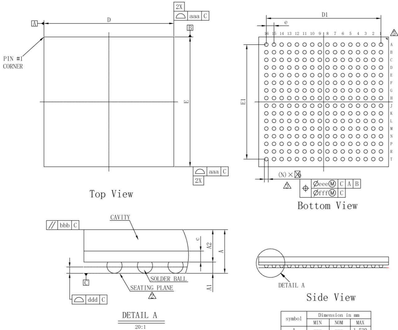
图 4-19 封装尺寸 PG256S/PG256
