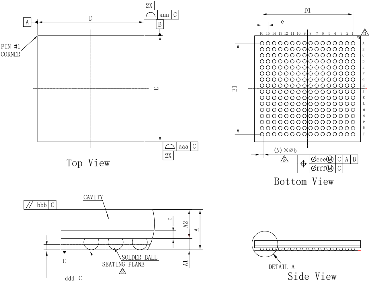
图 4-5 封装尺寸 UG256C
