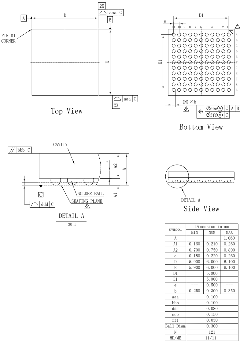
图 4-1 封装尺寸 MG121N
