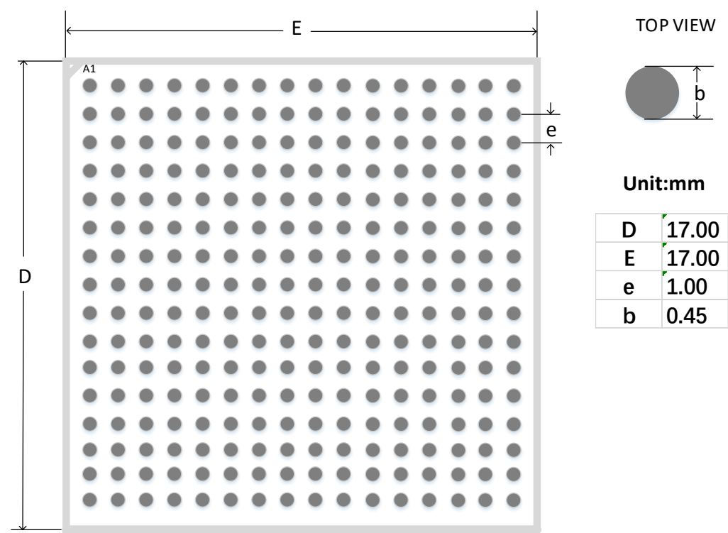
图 4-20 推荐 PCB Layout PG256S/PG256
