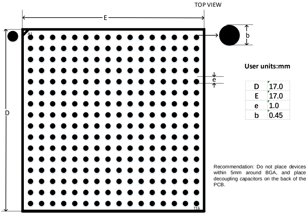
图 4-8 推荐 PCB Layout PG256C
