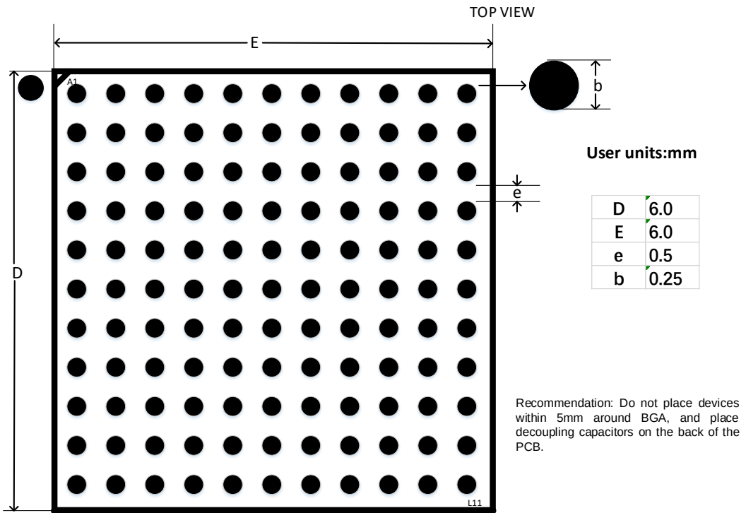
图 4-2 推荐 PCB Layout MG121N
