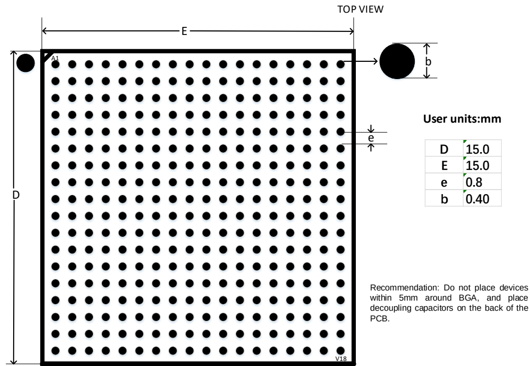
图 4-4 推荐 PCB Layout UG324S
