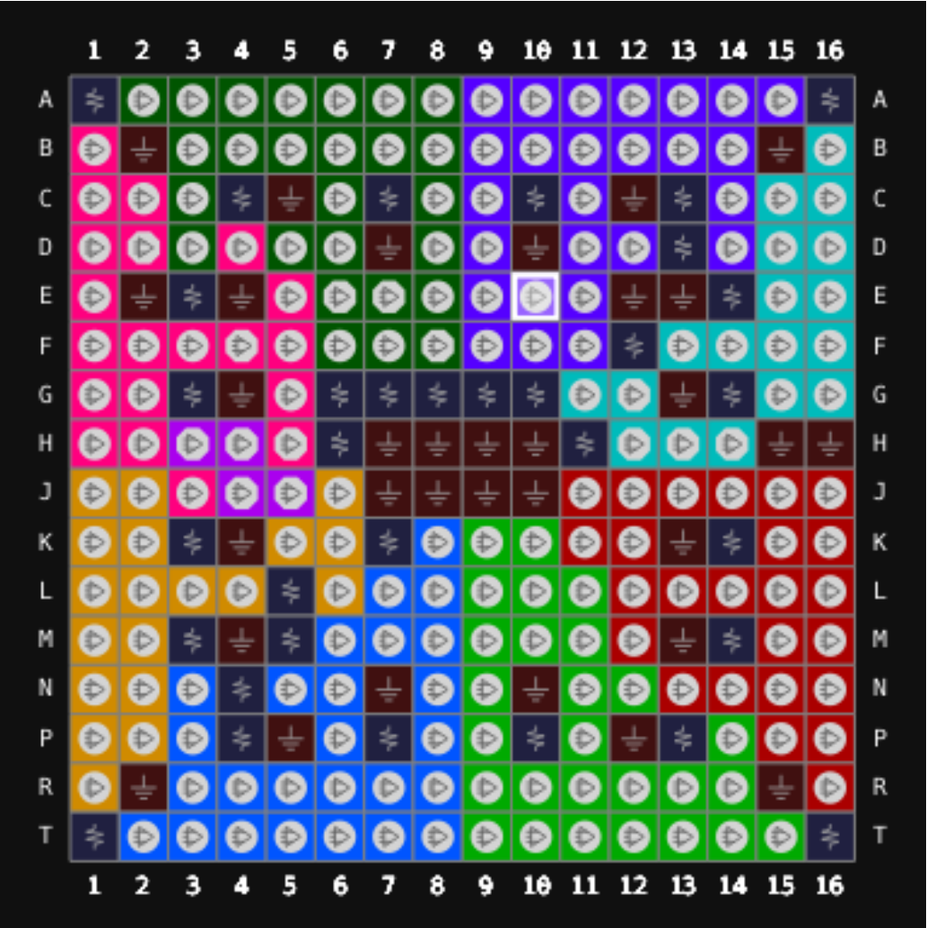
图 3-4 GW5A-25 器件 PG256C EV 版本封装管脚分布示意图（顶视图）
