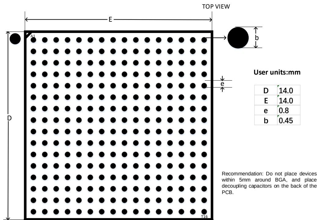
图 4-6 推荐 PCB Layout UG256C
