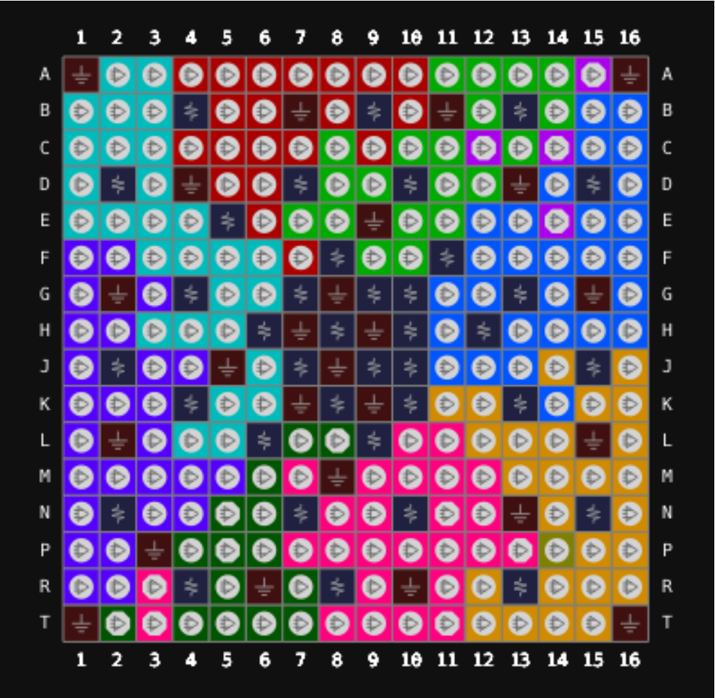
图 3-12 GW5A-25 器件 PG256S EV 版本封装管脚分布示意图（顶视图）
