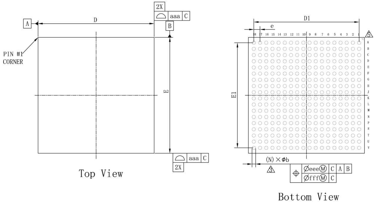
图 4-29 封装尺寸 UG324S
