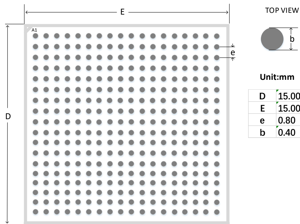
图 4-28 推荐 PCB Layout UG324A
