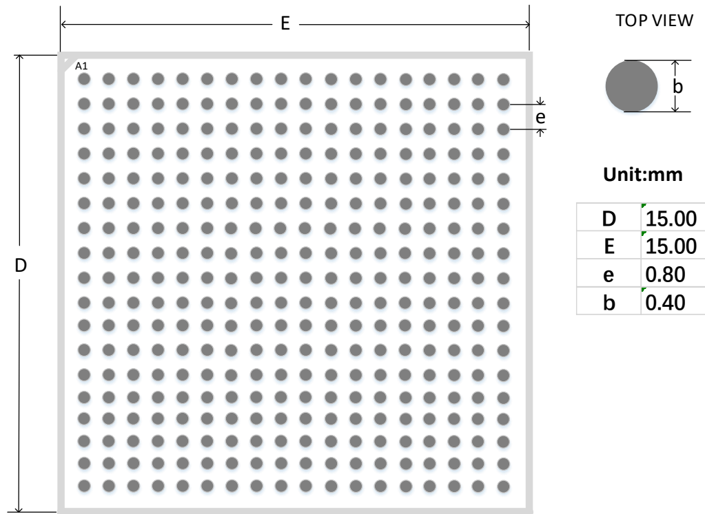
图 4-30 推荐 PCB Layout UG324S
