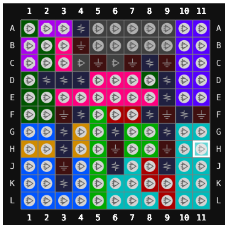
图 3-1 GW5A-25 器件 MG121N 封装管脚分布示意图（顶视图）
