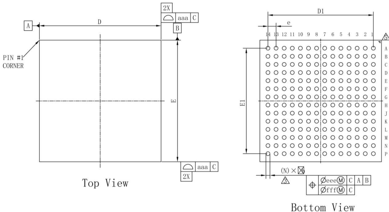
图 4-23 封装尺寸 PG196S
