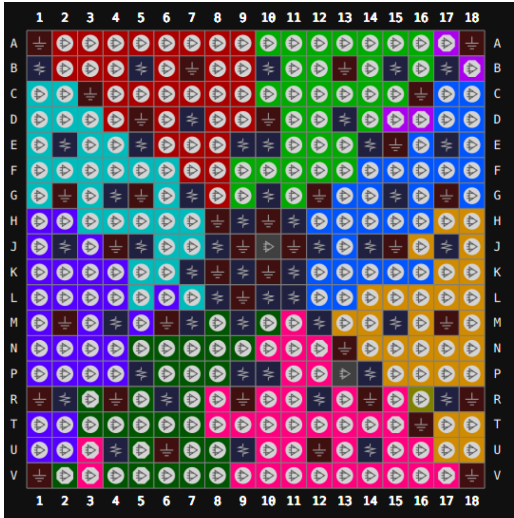
图 3-3 GW5A-25 器件 UG324S LV 版本封装管脚分布示意图（顶视图）
