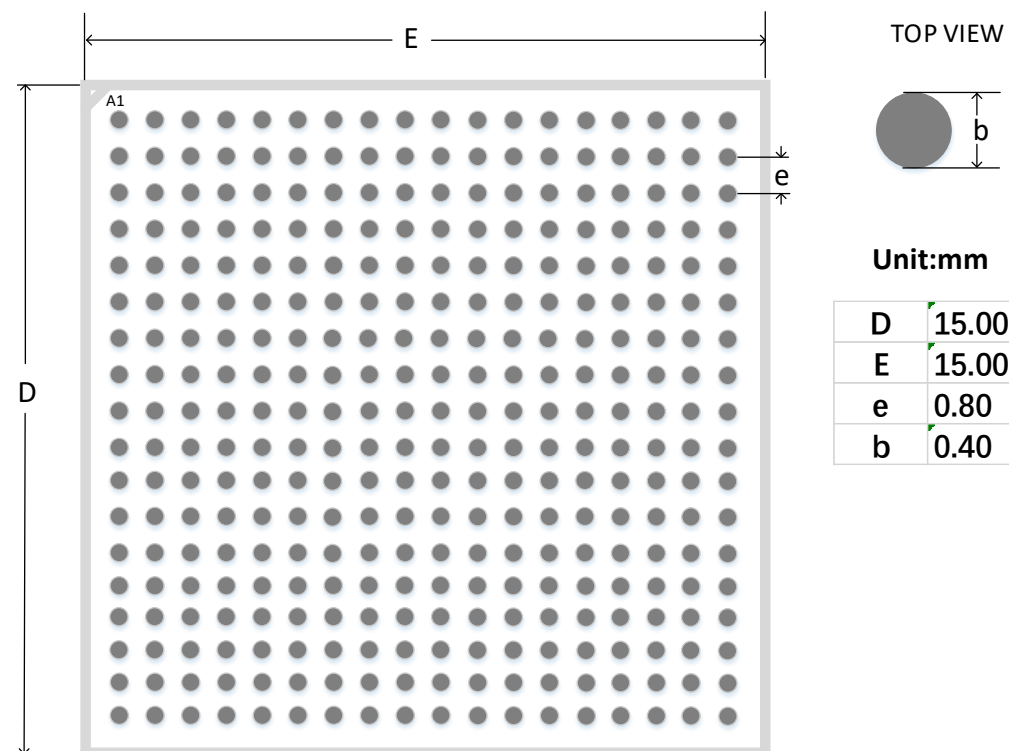
图 4-24 推荐 PCB Layout UG324A
