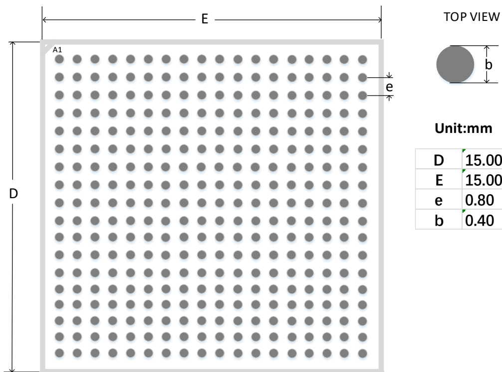
图 4-22 推荐 PCB Layout UG324
