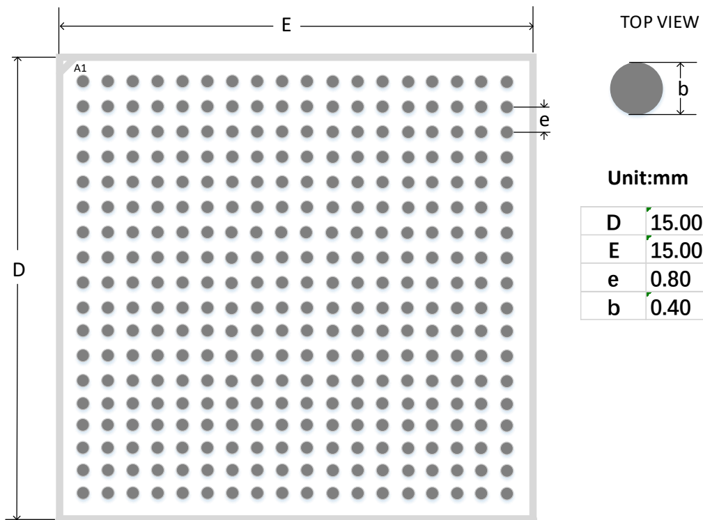
图 4-32 推荐 PCB Layout UG324S
