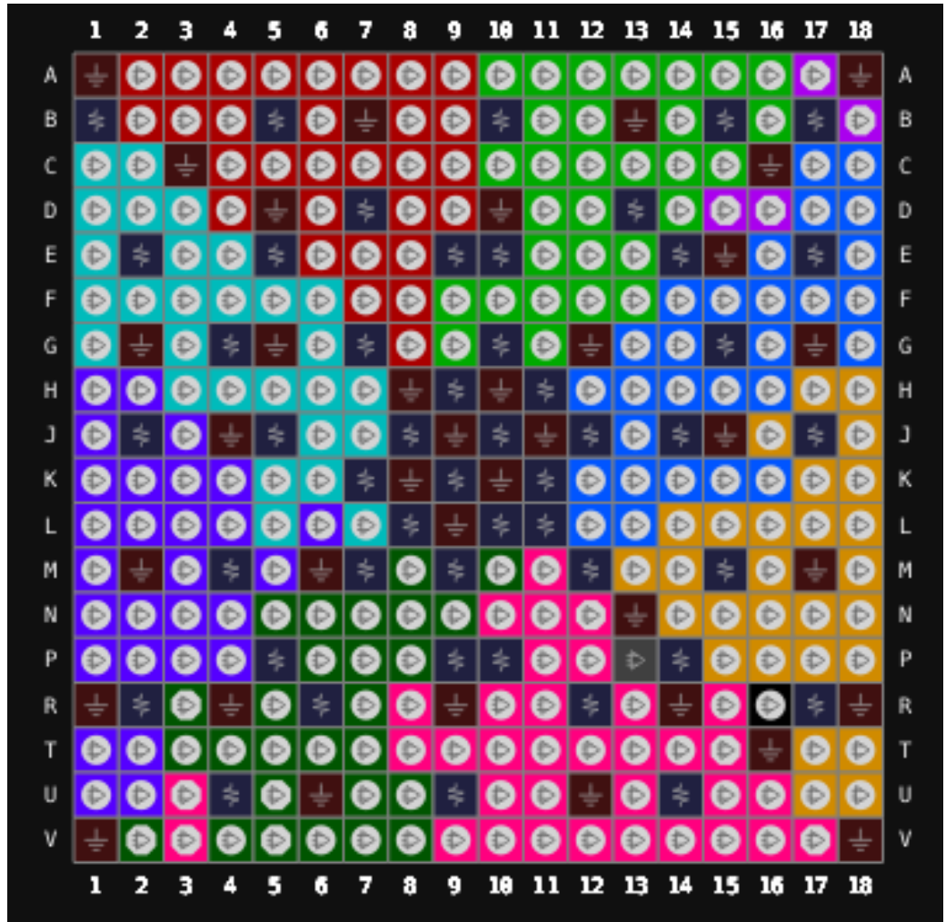
图 3-16 GW5A-25 器件 UG324S EV 版本封装管脚分布示意图（顶视图）
