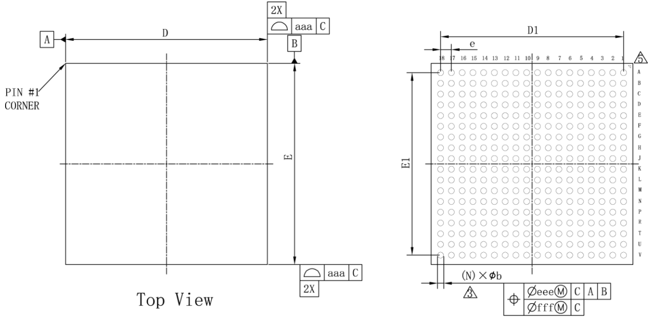
图 4-31 封装尺寸 UG324S
