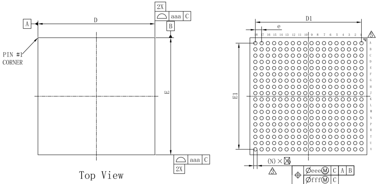
图 4-27 封装尺寸 UG324F
