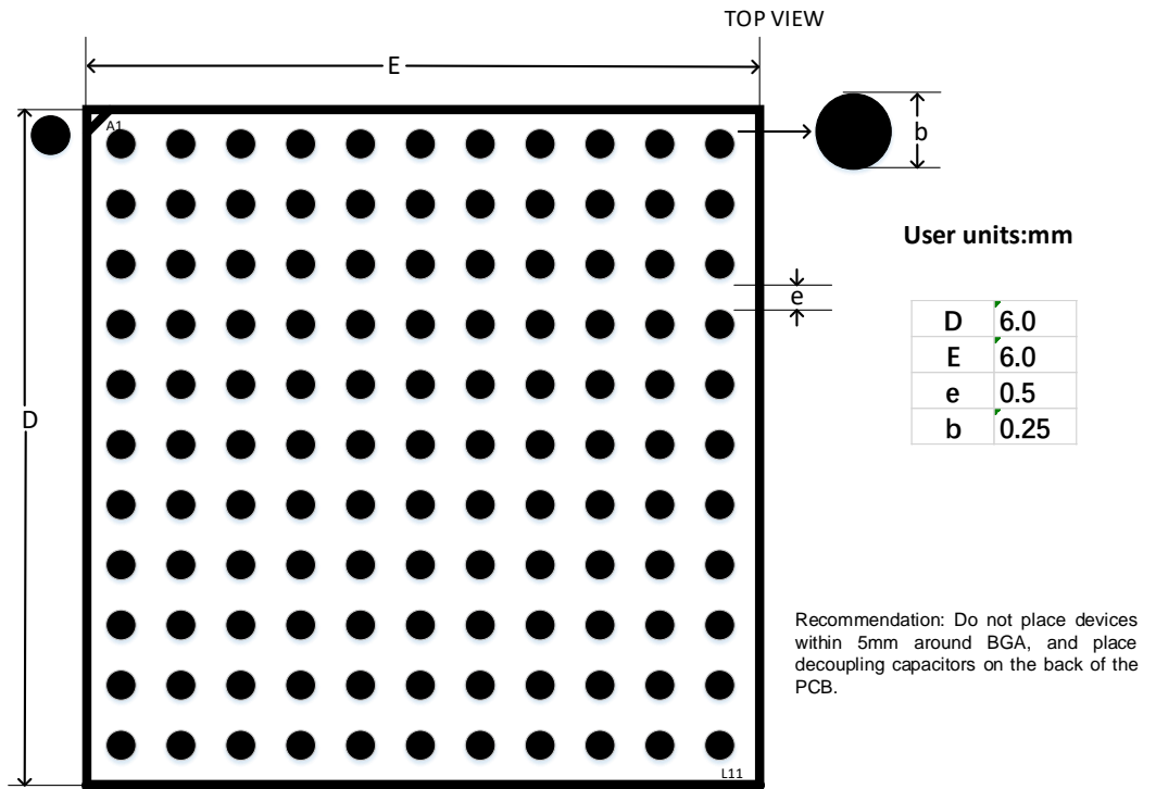
图 4-6 推荐 PCB Layout MG121N
