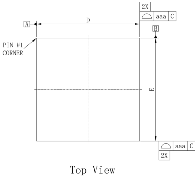
图 4-17 封装尺寸 UG225S
