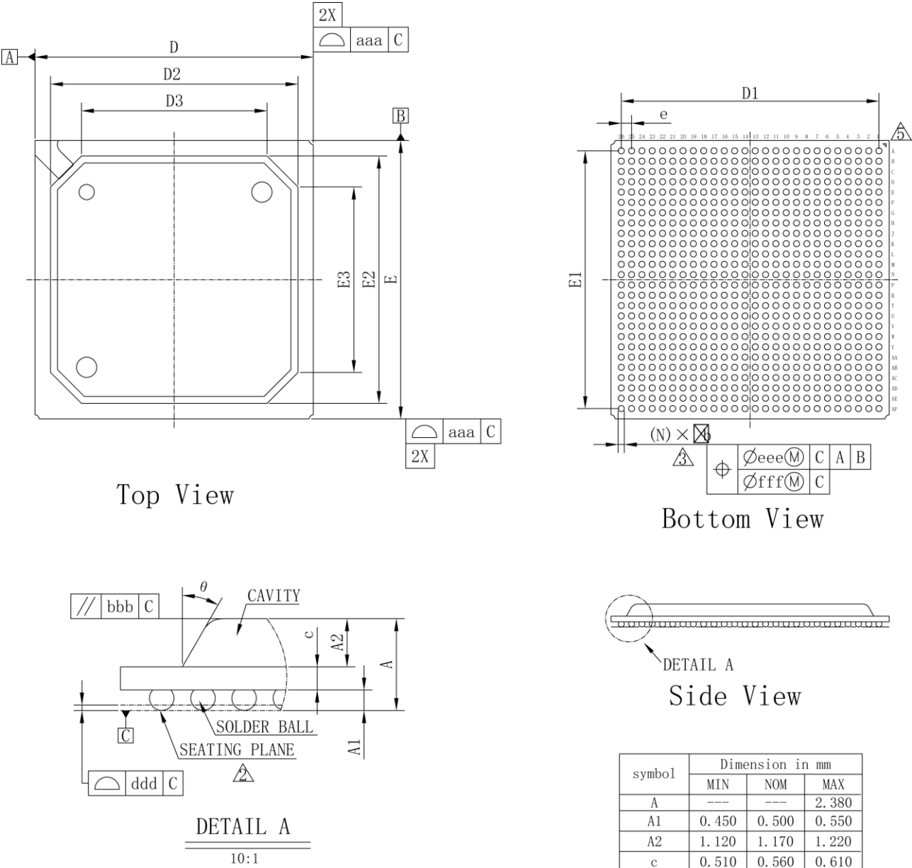
图 4-5 封装尺寸 PG676A
