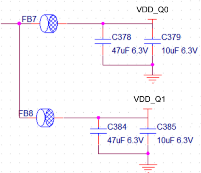
图 2-2 磁珠隔离
