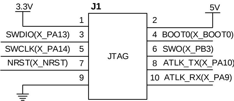
图 4-9 MCU AT-Link 接口连接示意图
