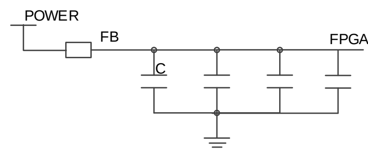
图 2-1 隔离滤波
