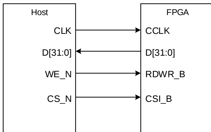
图 4-7 CPU 配置模式连接示意图
