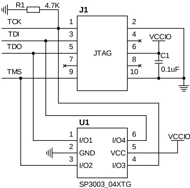
图 4-1 JTAG 配置模式连接示意图
