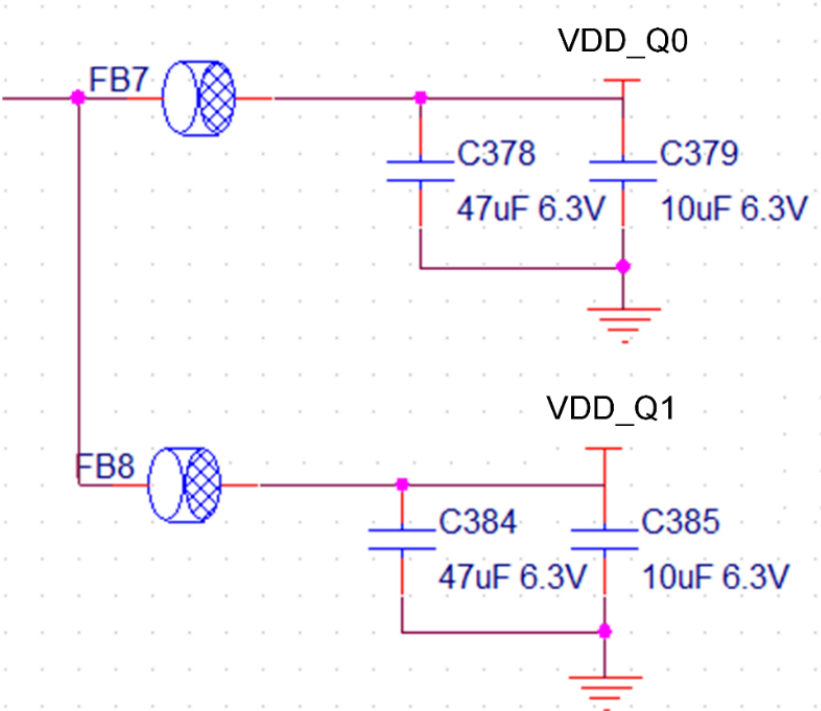
图 2-2 磁珠隔离
