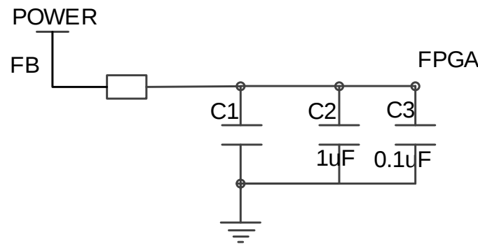
图 2-1 隔离滤波
