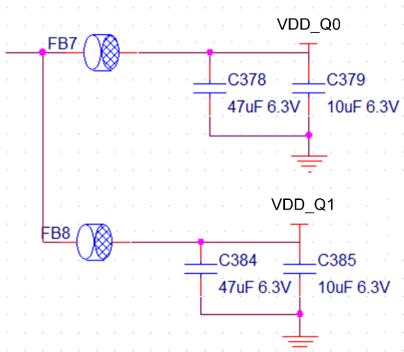
图 2-2 磁珠隔离
