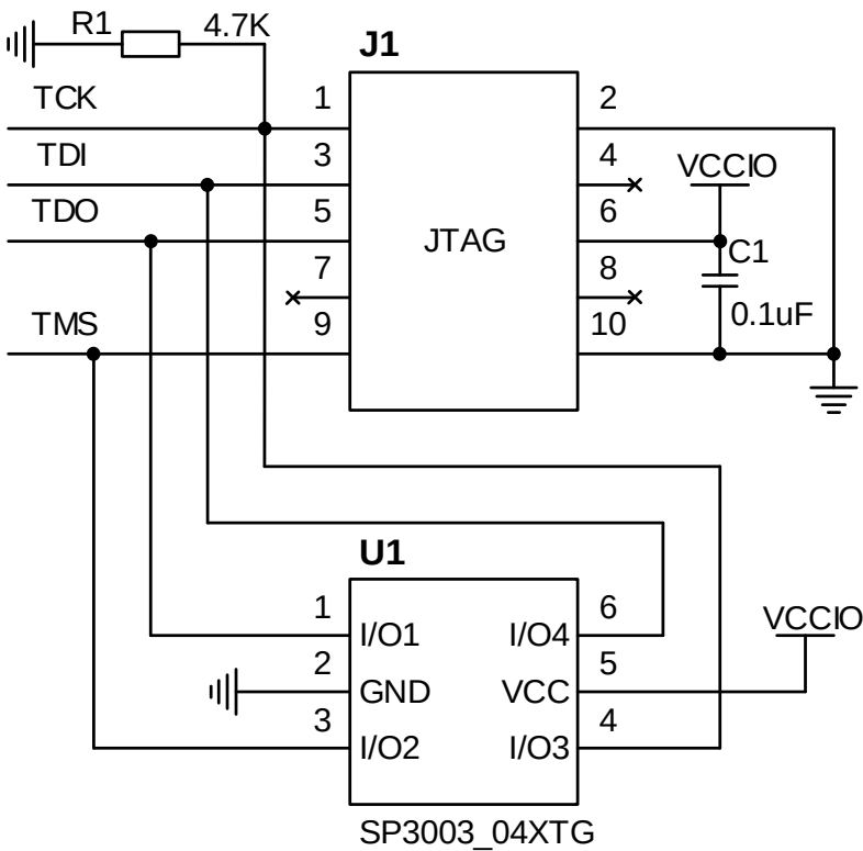
图 4-1 JTAG 配置模式连接示意图
