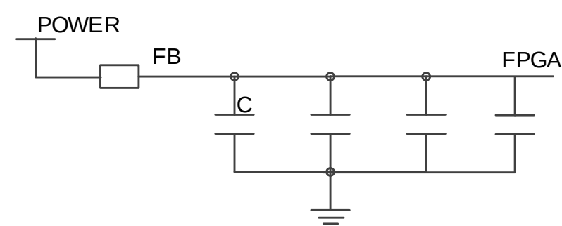
图 2-1 隔离滤波
