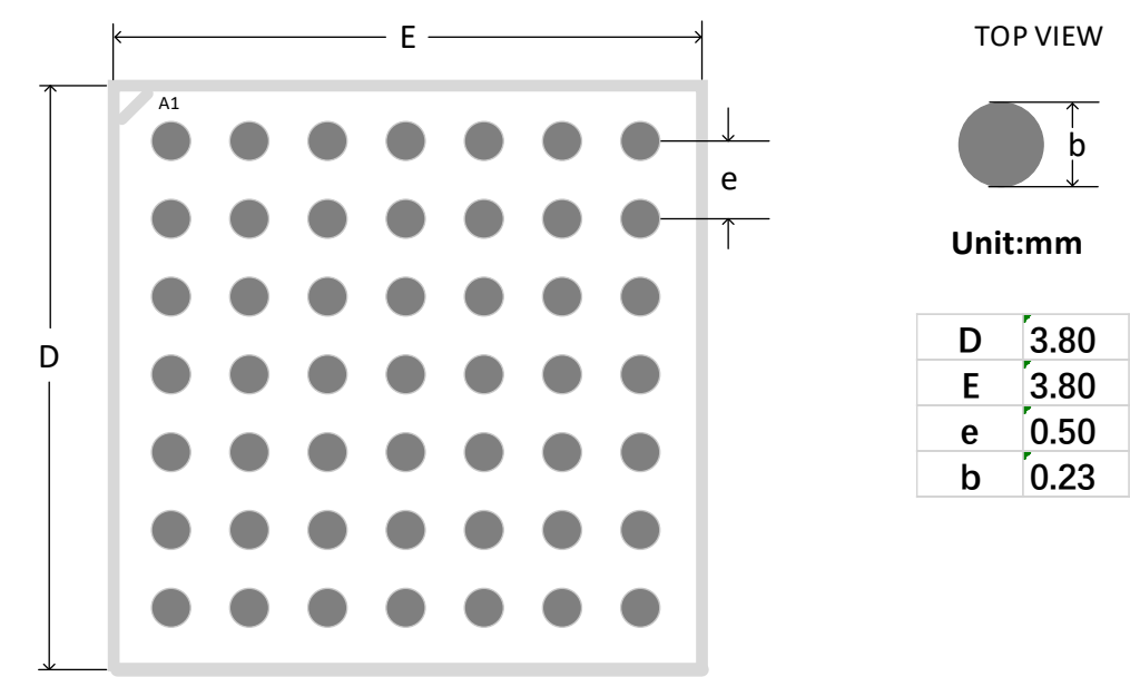
图 4-6 推荐 PCB Layout MG49P/MG49PG/MG49G
