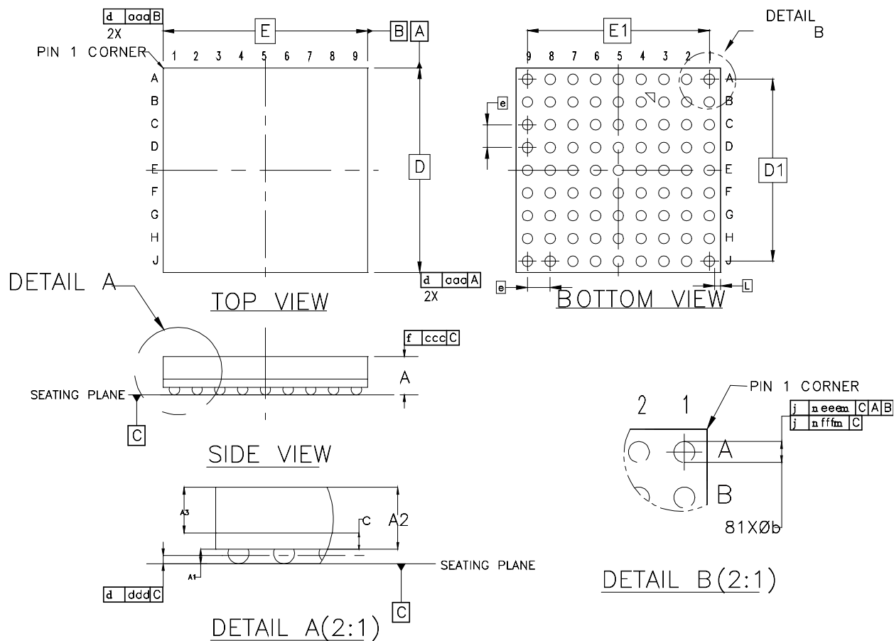
图 4-7 封装尺寸 MG81P
