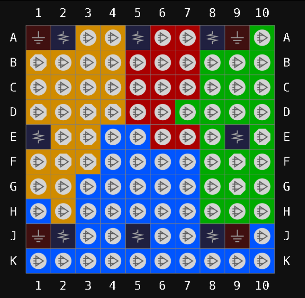
图 3-14 GW1NR-9 器件 MG100PT 封装管脚分布示意图（顶视图）
