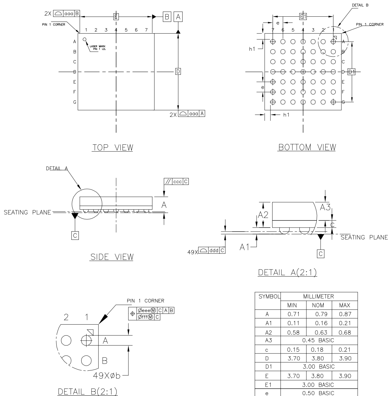
图 4-5 封装尺寸 MG49P/ MG49PG/MG49G
