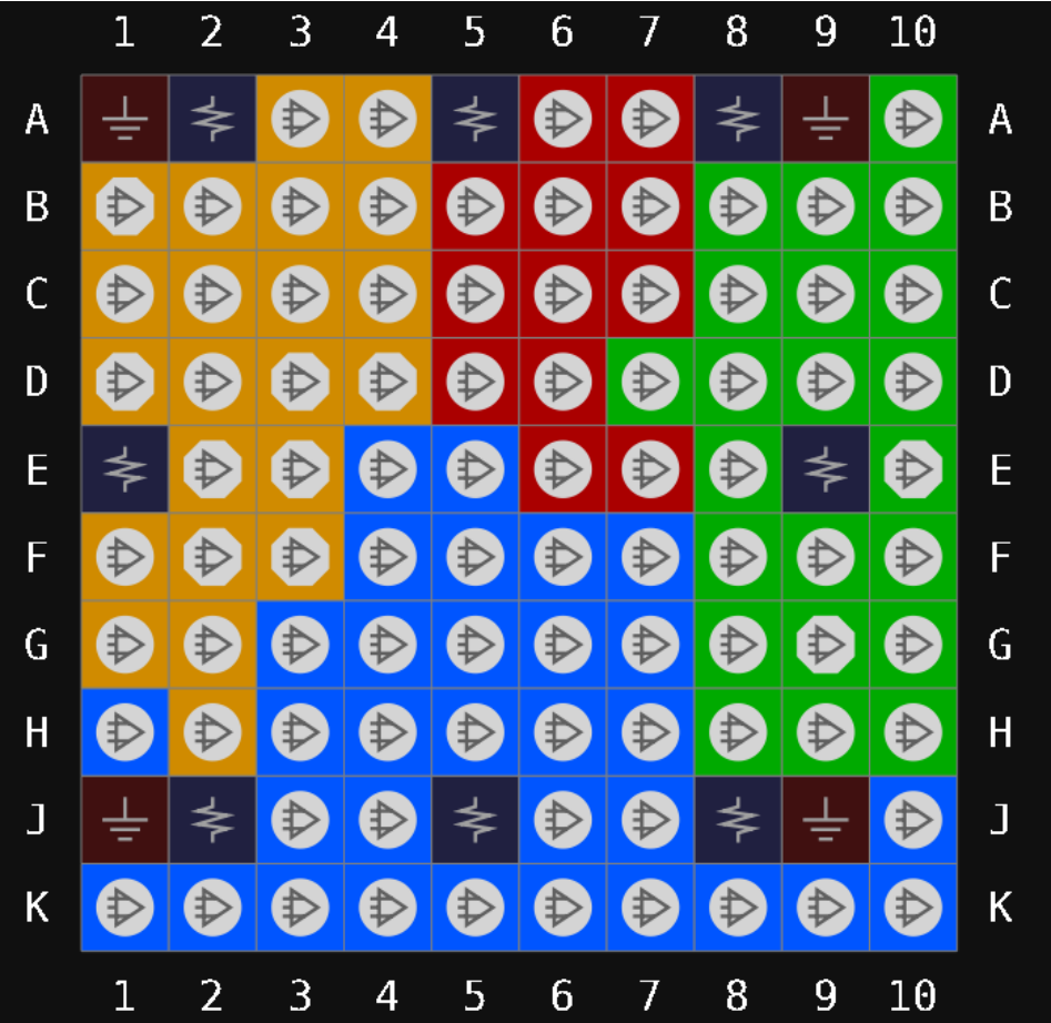
图 3-12 GW1NR-9 器件 MG100PA 封装管脚分布示意图（顶视图）
