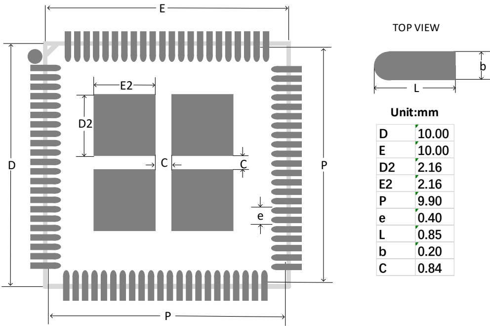
图 4-2 推荐 PCB Layout QN88/QN88P
