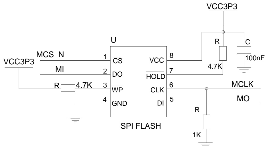
图 4 MSPI 电路
