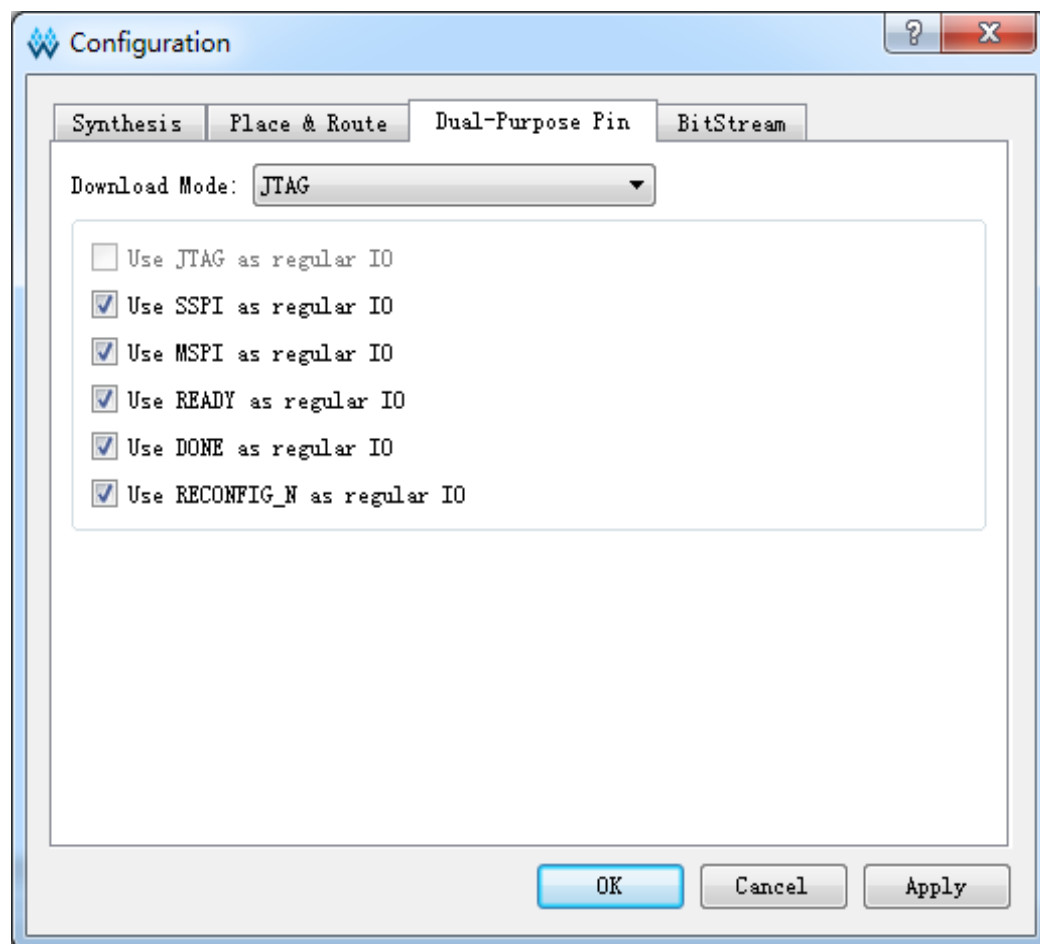
图 7 配置管脚复用
