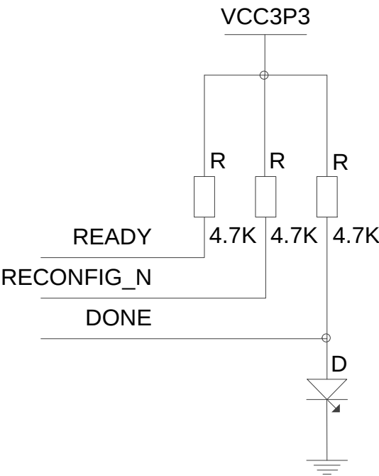
图 6 READY 、 RECONFIG_N 、 DONE 参考电路
