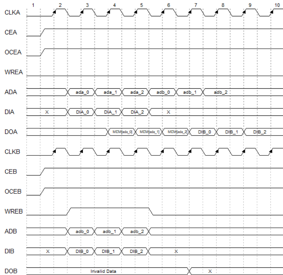
図 3-4 DPB/DPX9B Normal 書き込みモード(ポート B は書き込み、ポート A は読み出し)のタイミング図 (Pipeline 読み出しモード)
