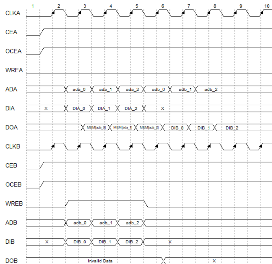
図 3-2 DPB/DPX9B Normal 書き込みモード(ポート B は書き込み、ポート A は読み出し)のタイミング図 (Bypass 読み出しモード)
