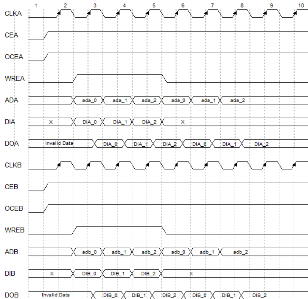
図 3-5 DPB/DPX9B Write-through 書き込みモードのタイミング図 (Bypass 読み出しモード)
