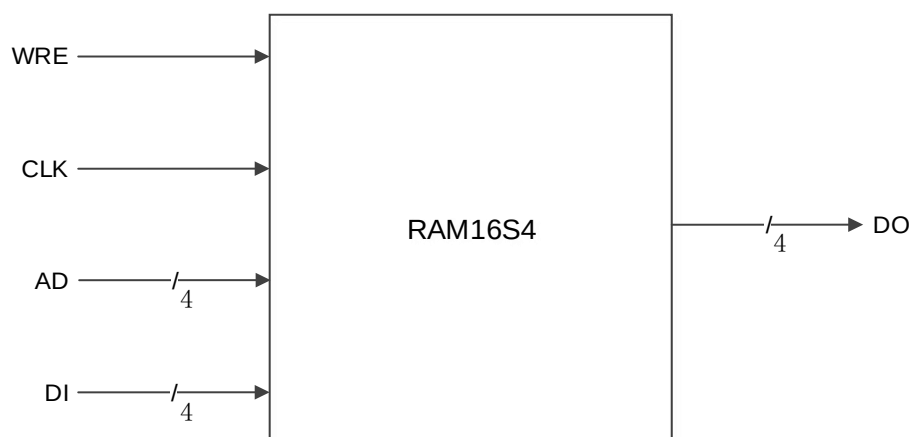
図 5-4 RAM16S4 のポート図
