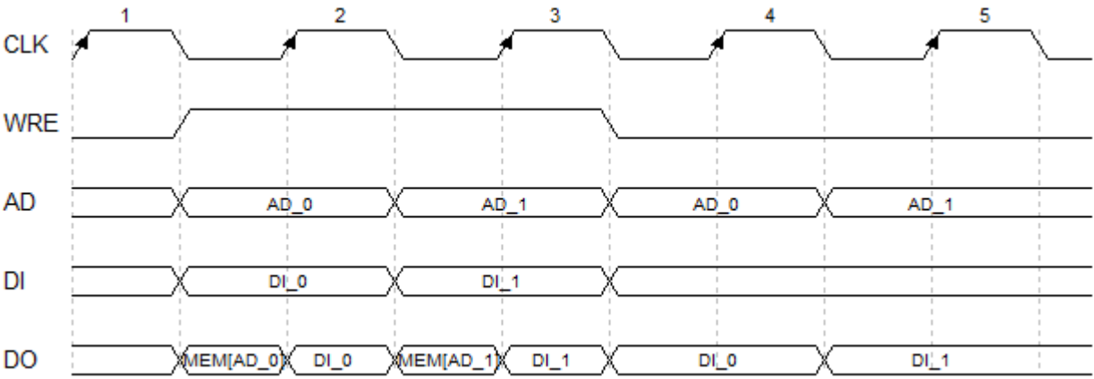
図 5-1 RAM16S1 モードのタイミング図
