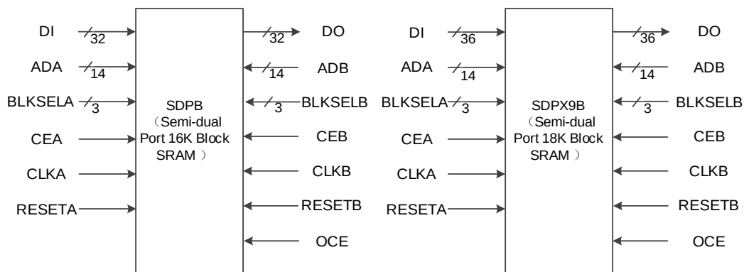
図 3-13 SDPB/SDPX9B のポート図
