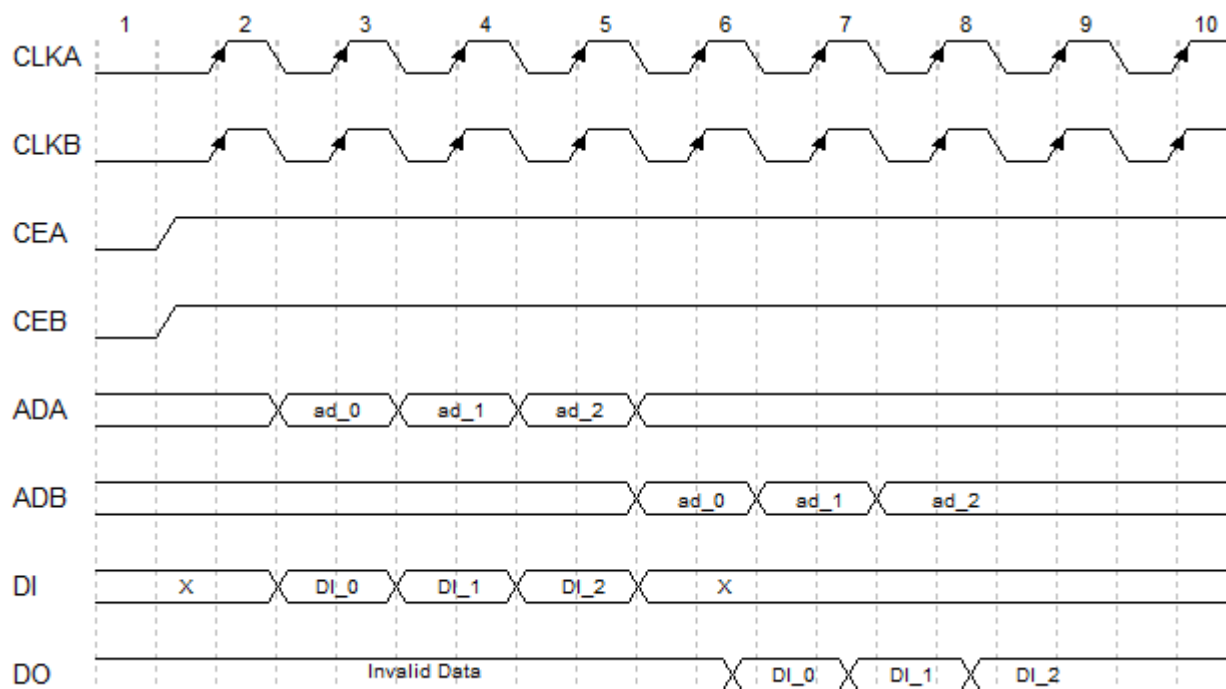
図 3-11 セミ・デュアル・ポート BSRAM Normal 書き込みモードのタイミング図 (Bypass 読み出しモード)
