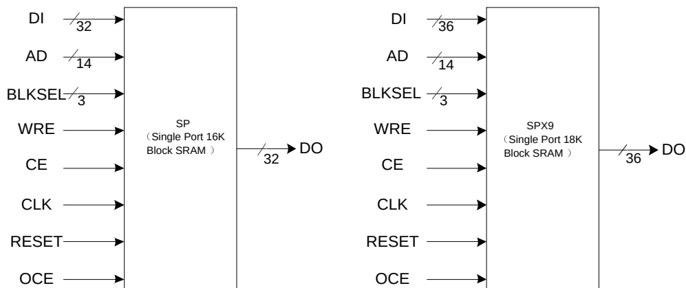
図 3-10 SP/SPX9 のポート図
