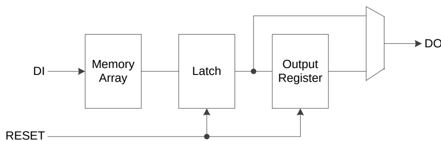
図 4-1 出力リセットのブロック図
