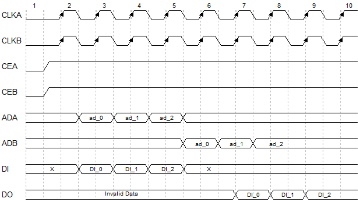
図 3-12 セミ・デュアル・ポート BSRAM Normal 書き込みモードのタイミング図 (Pipeline 読み出しモード)
