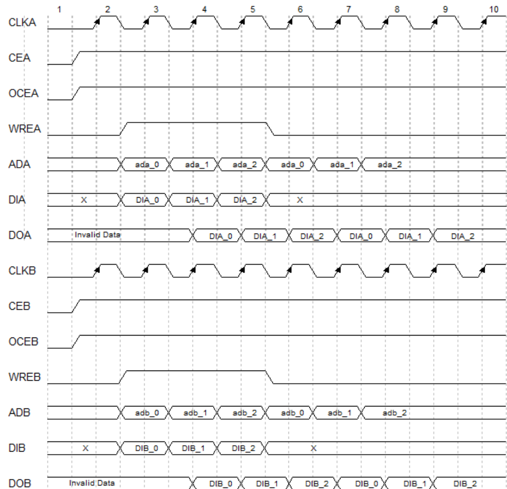
図 3-6 DPB/DPX9B Write-through 書き込みモードのタイミング図 (Pipeline 読み出しモード)
