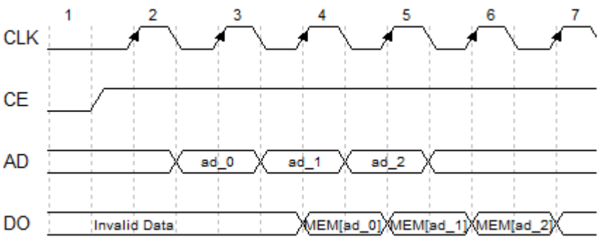
図 3-15 ROM のタイミング図 (Pipeline モード)
