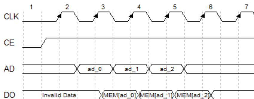
図 3-14 ROM のタイミング図 (Bypass モード)
