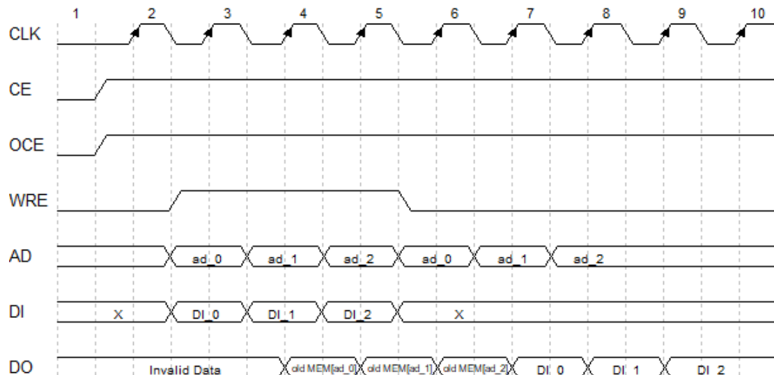
図 3-9 SP/SPX9 read-before-write 書き込みモードのタイミング図 (Pipeline 読み出しモード)
