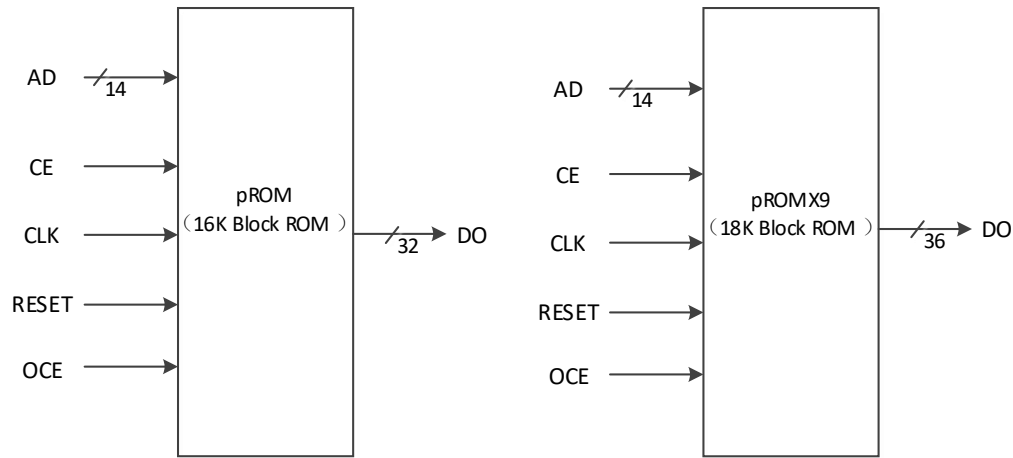
図 3-16 pROM/pROMX9 のポート図
