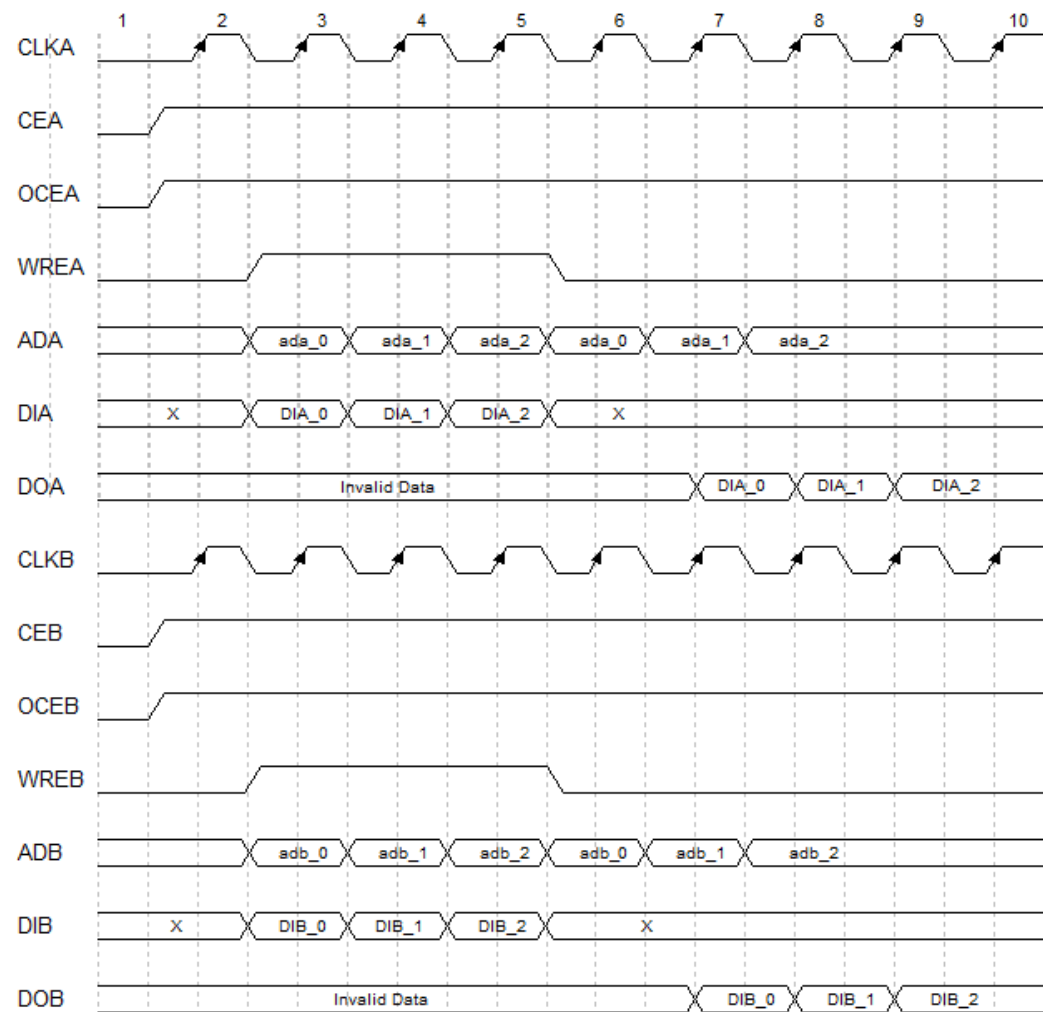
図 3-3 DPB/DPX9B Normal 書き込みモードのタイミング図 (Pipeline 読み出しモード)
