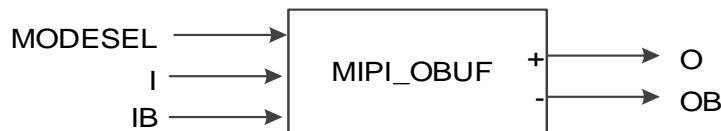
图 3-15 MIPI_OBUF 端口示意图
