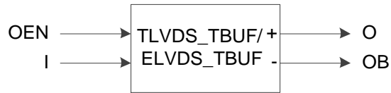
图 3-12 TLVDS_TBUF/ELVDS_TBUF 端口示意图
