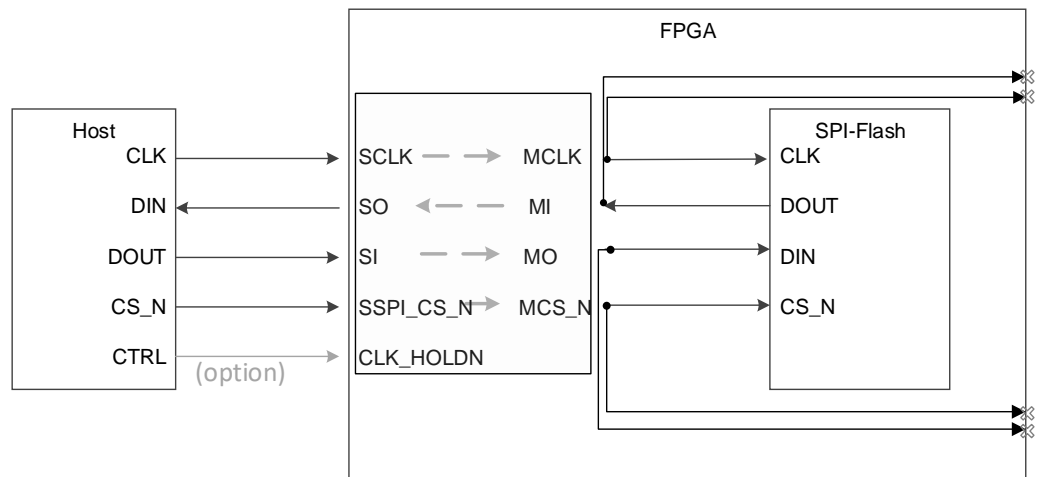
图 7-43 SSPI 编程内部 Flash 连接示意图(GW2ANR-18/GW2AN-55)
