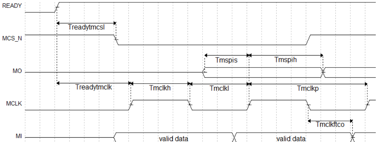
图 7-56 MSPI 下载模式时序图
