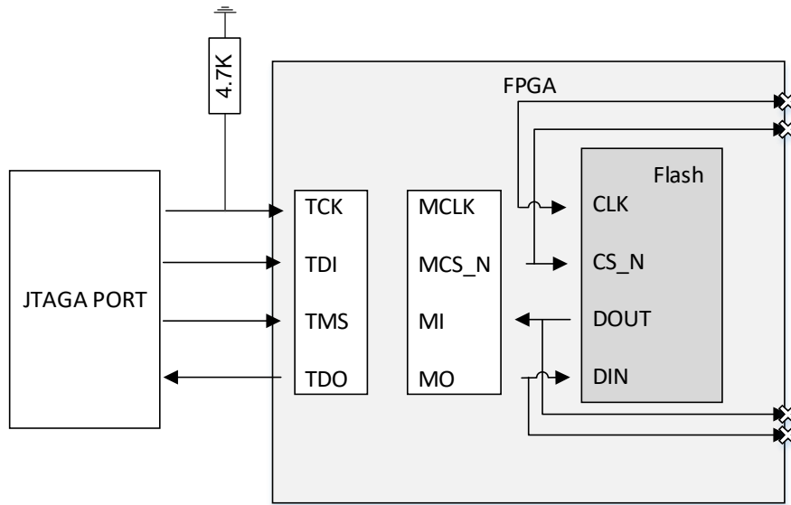
图 7-27 JTAG 接口编程内部 SPI-Flash 连接示意图 (GW2ANR-18/GW2AN-55)
