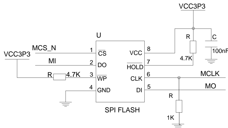
图 4 MSPI 电路参考
