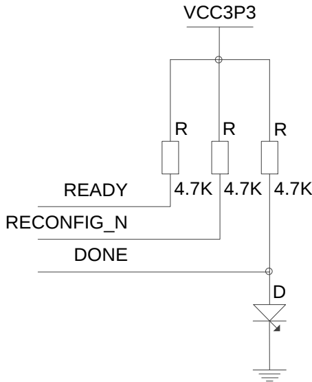
图 5 READY、RECONFIG_N、DONE 参考电路
