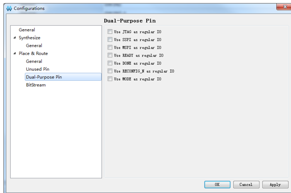
图 6 配置管脚复用
